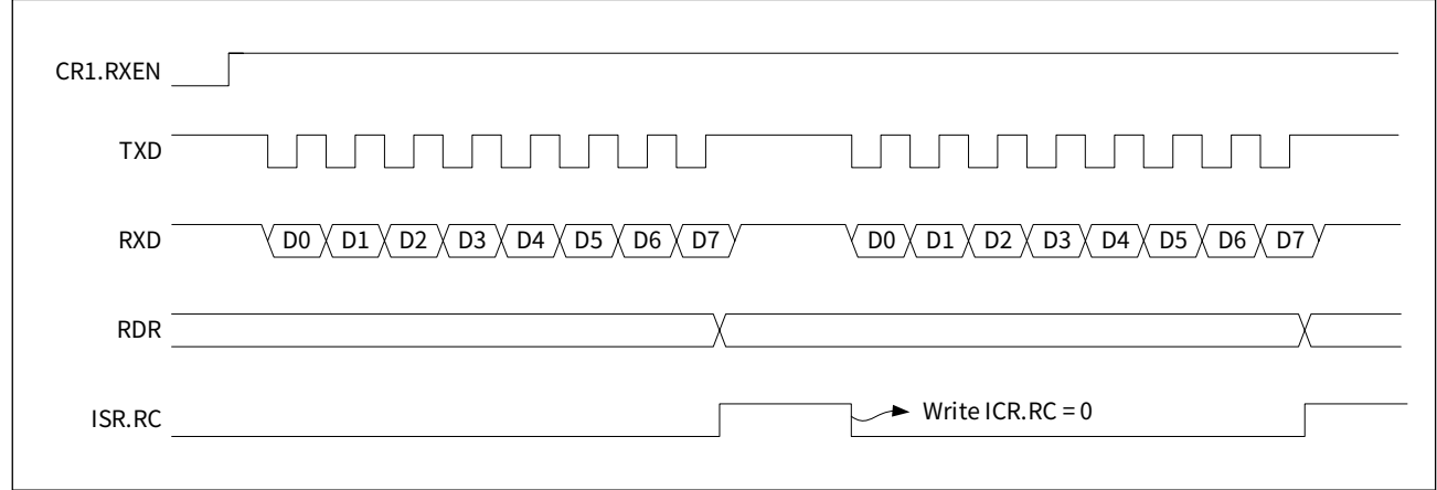
图 16-3 同步半双工模式接收时序（接收两个字节数据）
