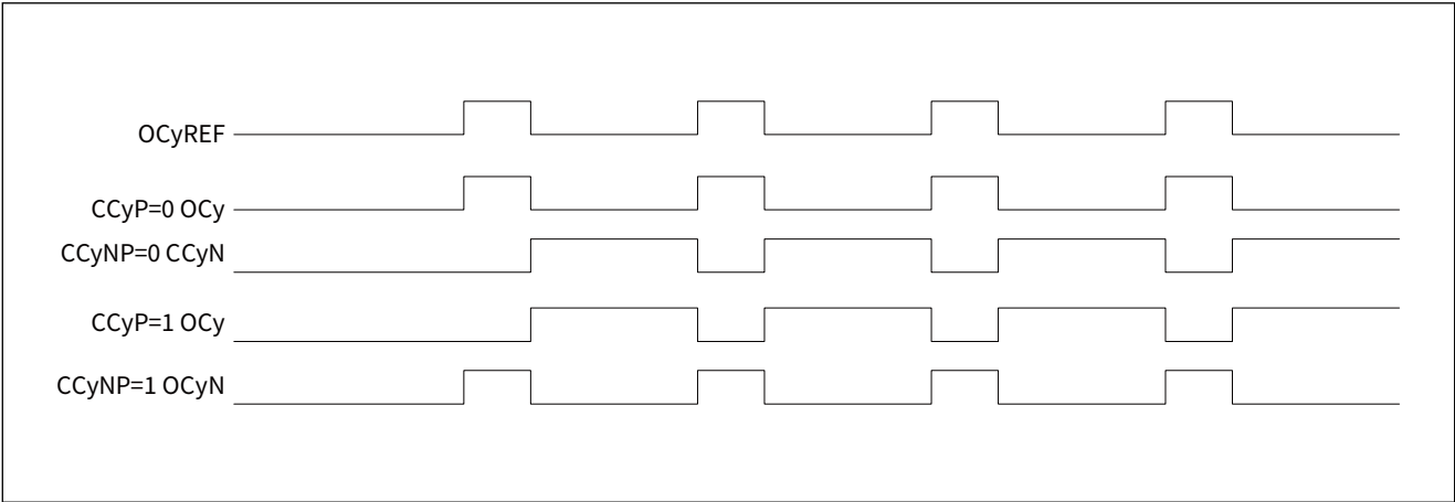
图 14-44 互补 PWM 输出波形
