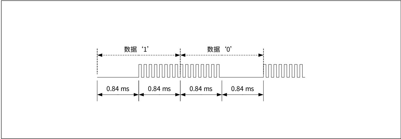
图 19-20 PPM 调制方式
