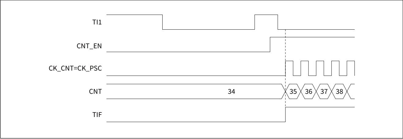
图 14-27 触发模式时序
