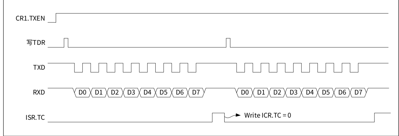
图 16-2 同步半双工模式发送时序（发送两个字节数据）
