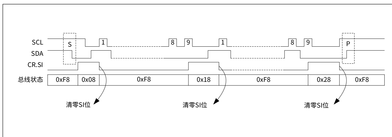
图 18-7 主机发送模式状态同步图
