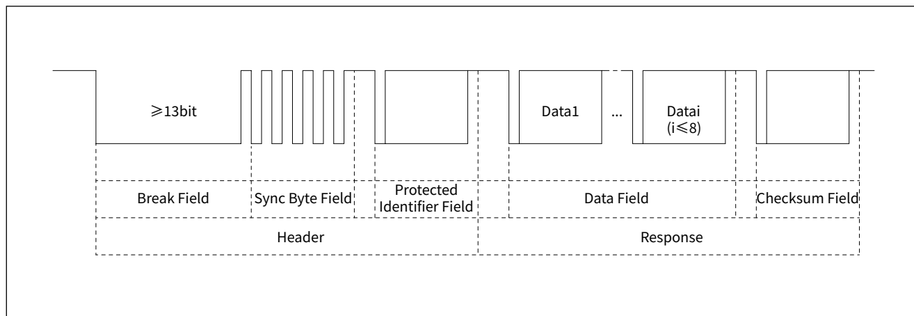
图 16-11 LIN 帧的结构
