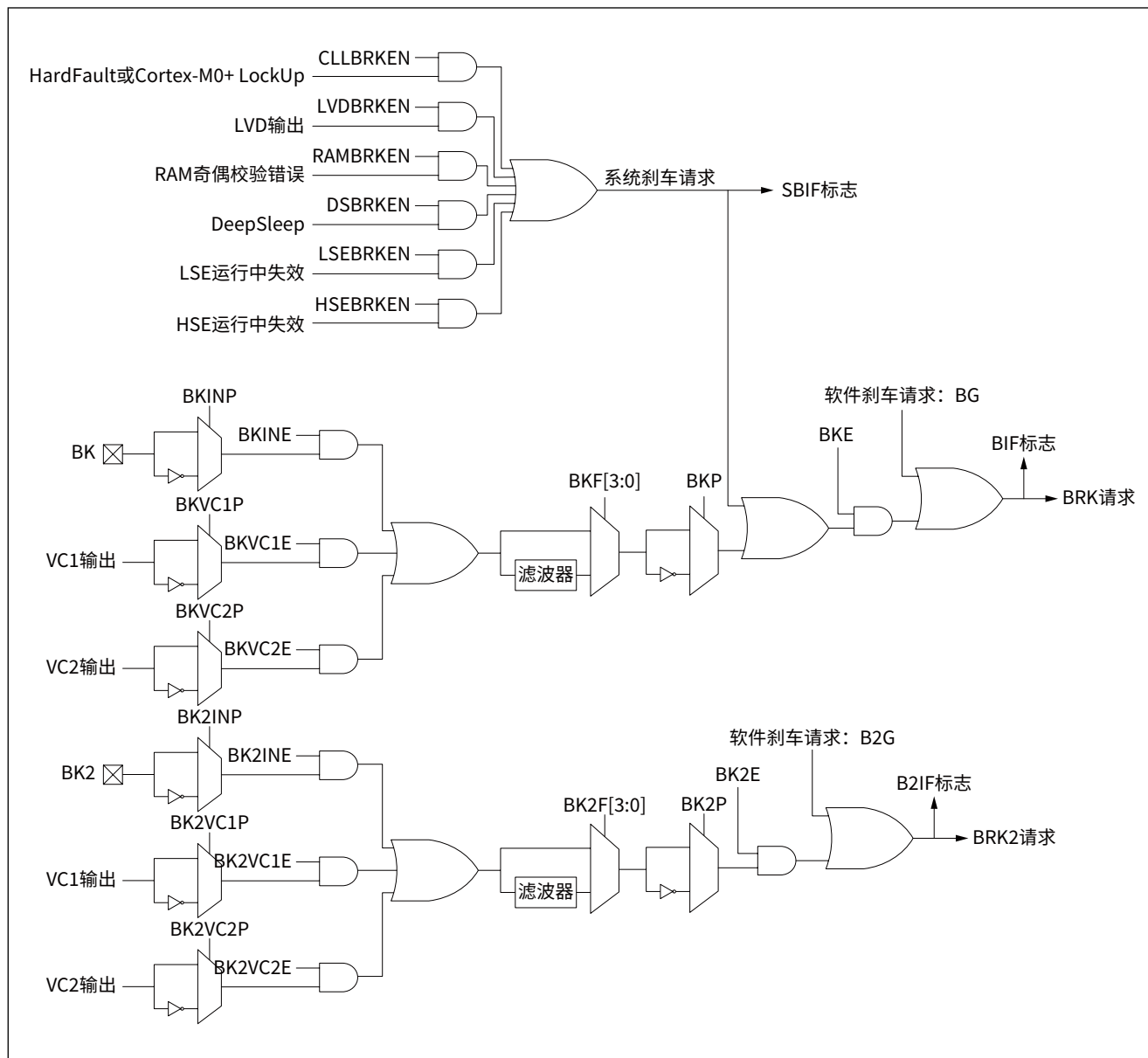
图 14-46 刹车和刹车 2 电路
