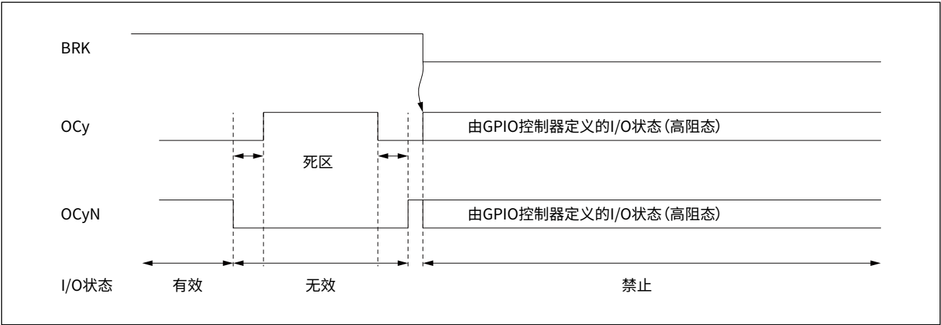
图 14-48 响应刹车事件 BRK 时的输出行为 (OSSI=0)
