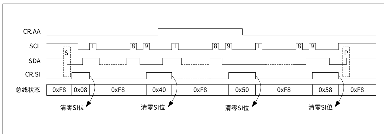
图 18-9 主机接收模式状态同步图
