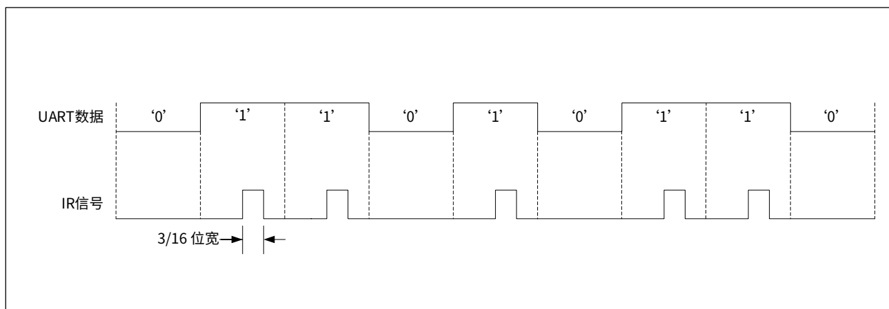
图 19-22 高速 UART 调制方式
