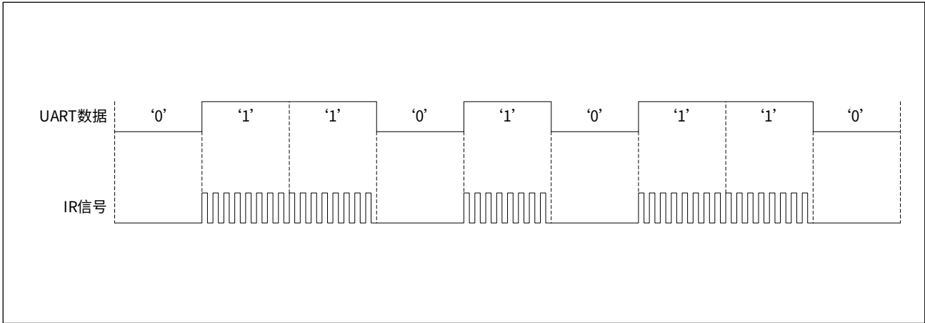
图 19-21 UART 调制方式
