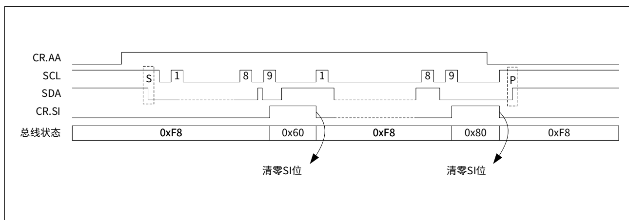
图 18-11 从机接收模式状态同步图
