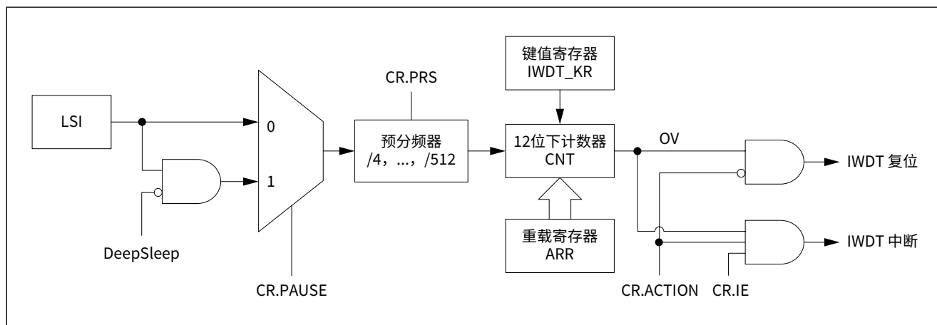
图 15-1 IWDT 功能框图
