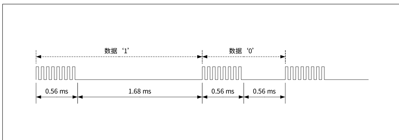
图 19-19 PWM 调制方式
