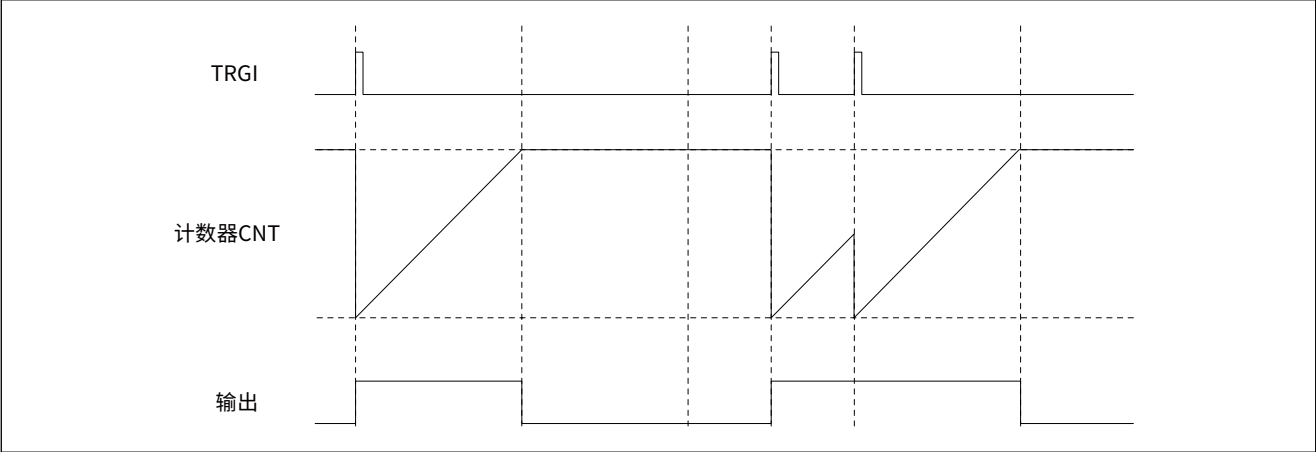
图 14-50 可再触发单脉冲模式 2 示例
