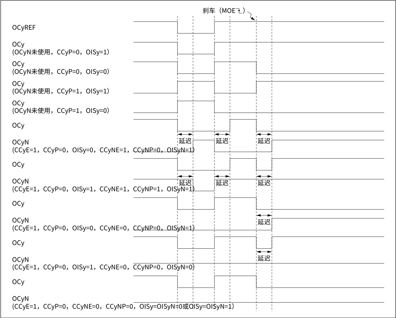
图 14-48 响应刹车事件 BRK 时的输出行为 (OSSI=0)
