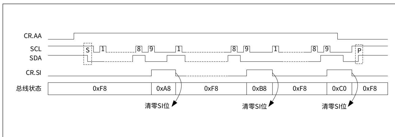
图 18-13 从机发送模式状态同步图
