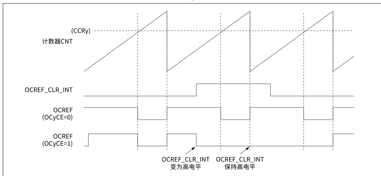
图 14-51 OCyREF 清零示例
