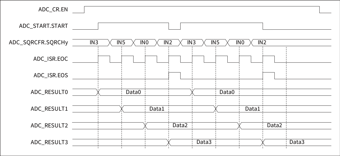
图 20-4 序列 1 扫描转换时序图
