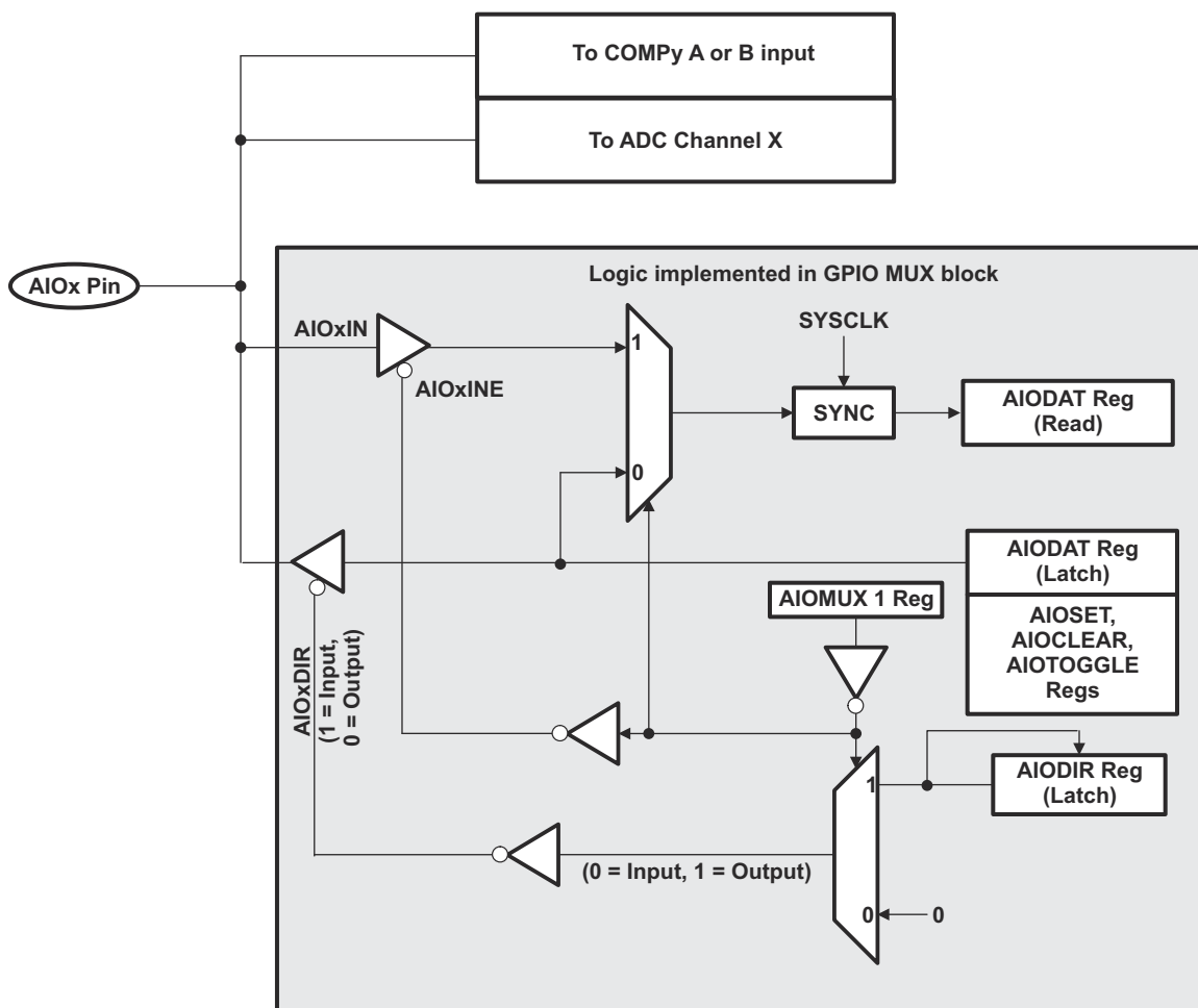
ADC 通道和比较器功能始终可用。数字 I/O 功能只有当 AIOMUX1 寄存器中的相应位为 0 时可用。在此模式下，读取 AIOPAT 寄存器会反映实际引脚状态。
