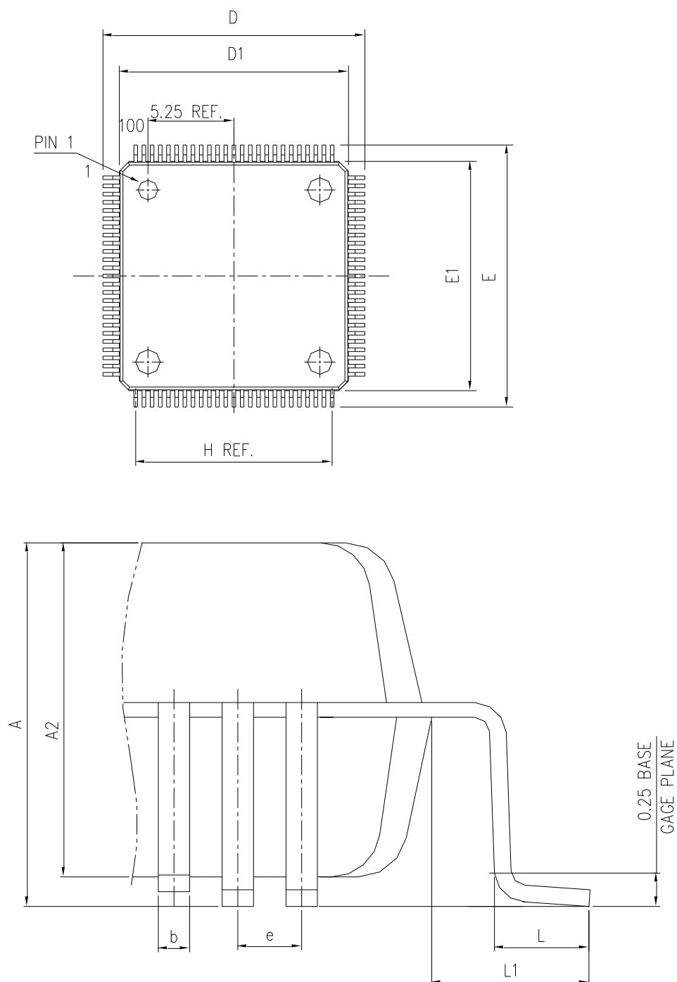
图 19 LQFP100 封装图
