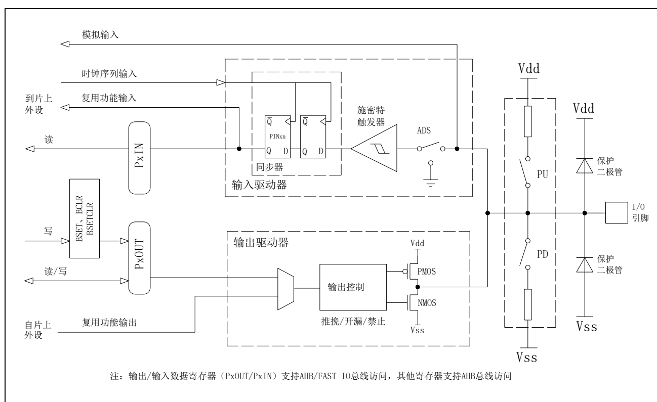
图 6-1 端口电路图
