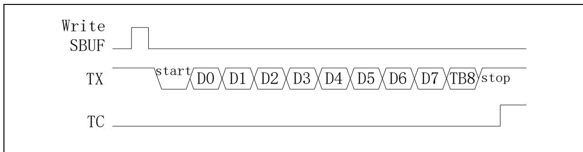
图 22-6 Mode2 发送数据
