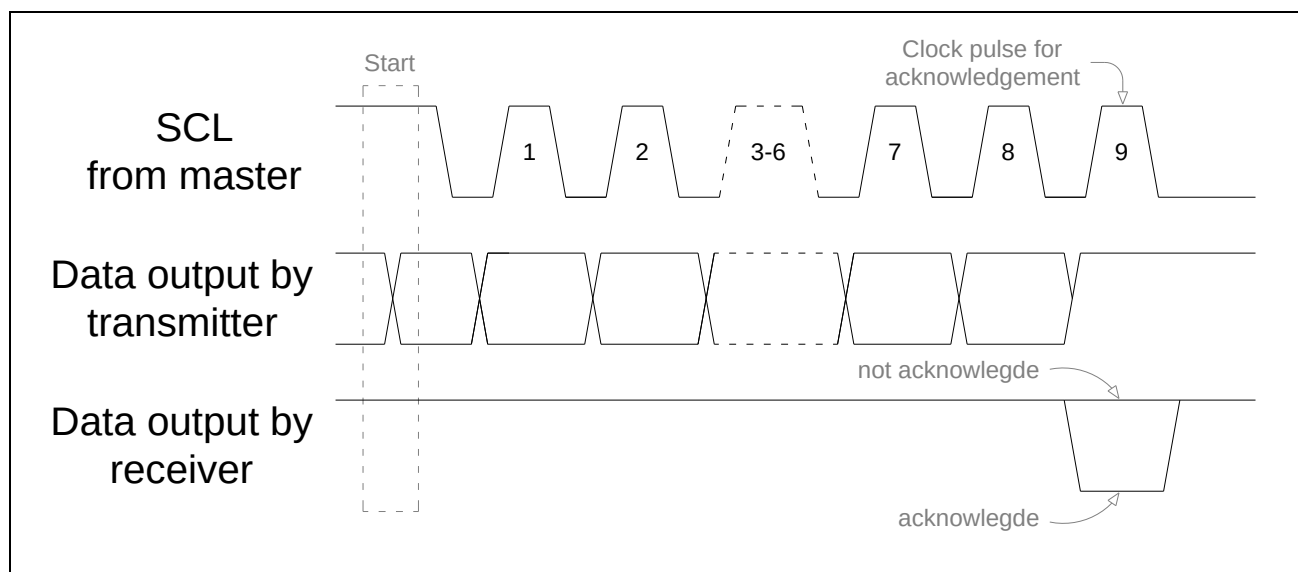
图 7-4 I2C 总线上应答信号
