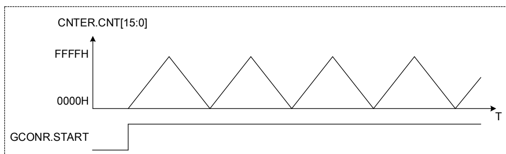
图 17-3 三角波波形
