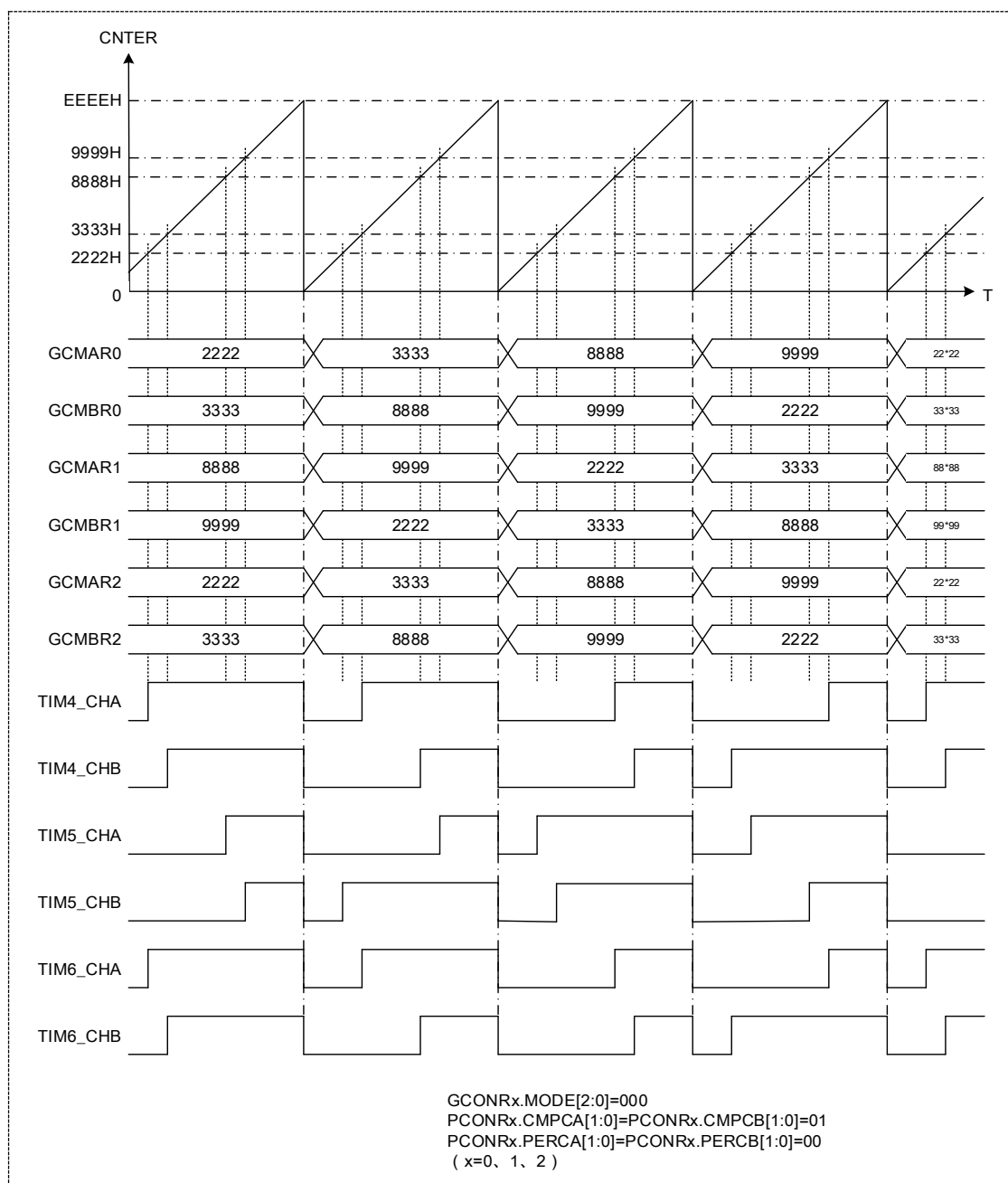
图 17-14 6 相 PWM 波
