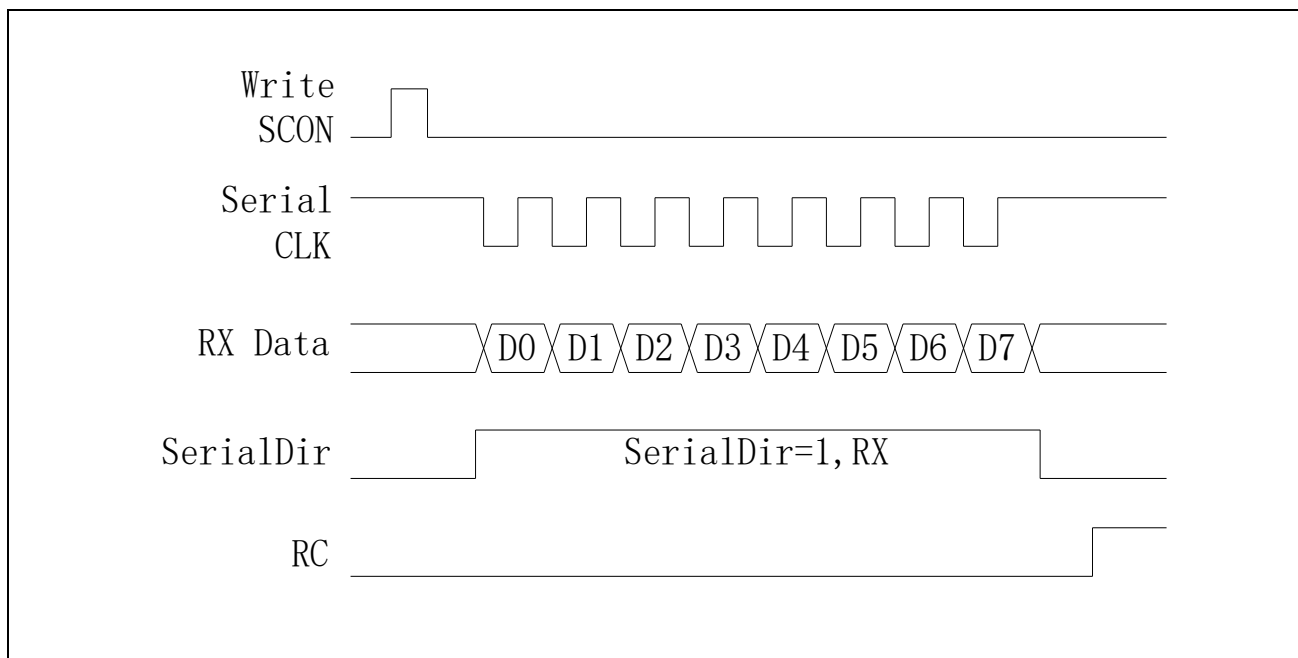
图 21-3 Mode0 接收数据
