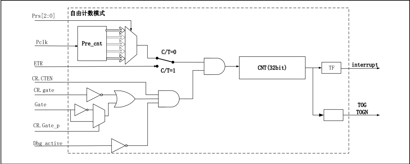
图 14-3 自由计数框图
