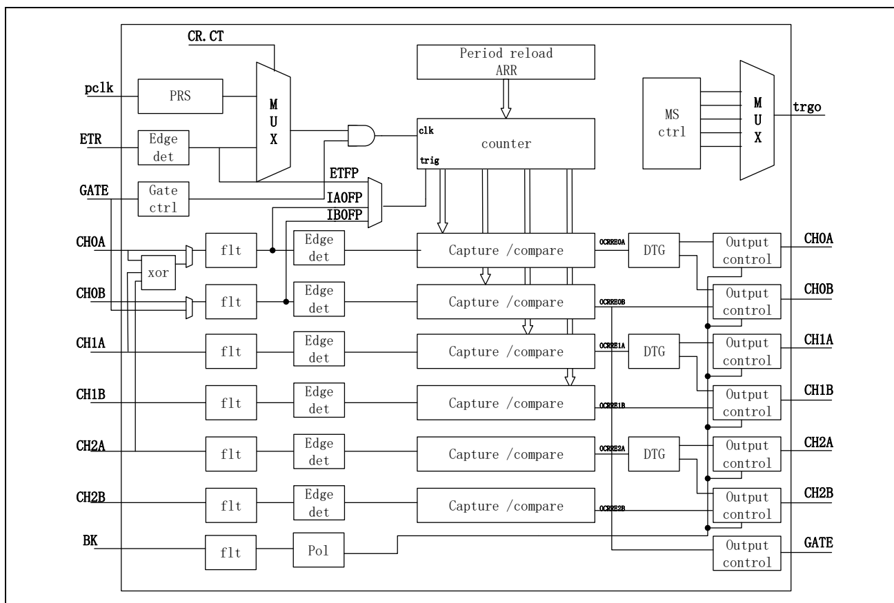
图 14-2 TIM3 框图
