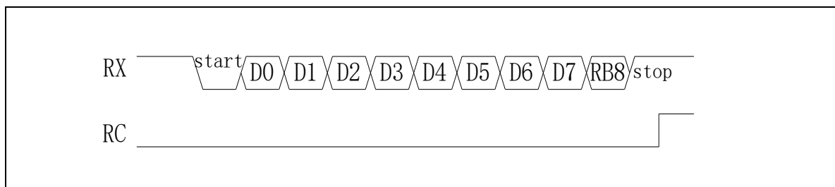
图 22-7 Mode2 接收数据
