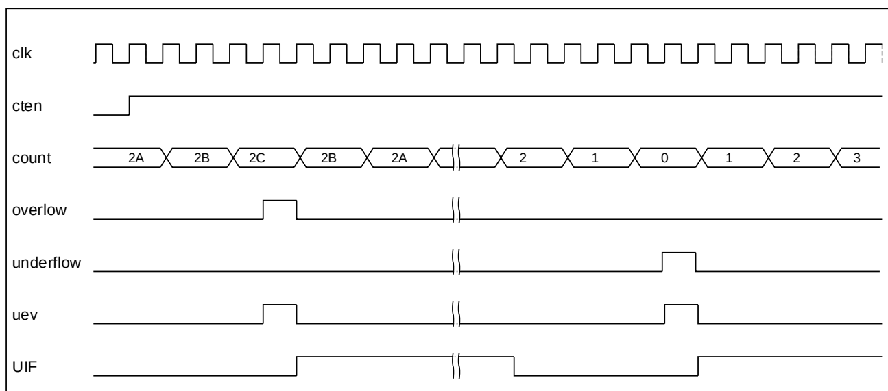
图 14-19 带预分频的上下计数
