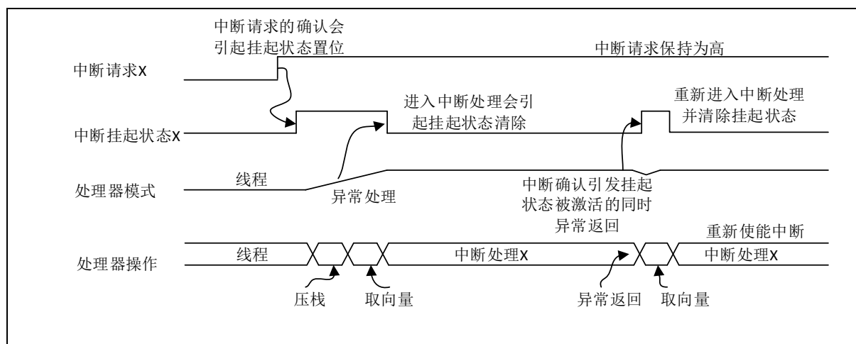
图 5-5 中断退出时若中断请求保持高电平就会引起中断处理的再次执行
