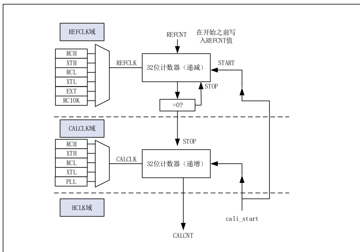
图 3-4 时钟校准原理图
