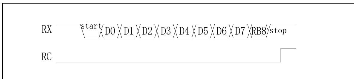
图 22-9 Mode3 接收数据
