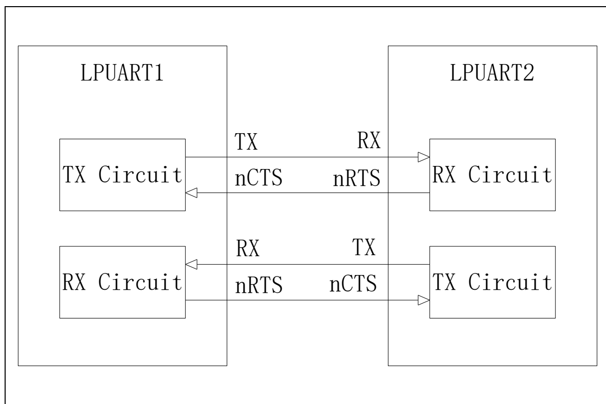
图 22-10 LPUART 硬件流控
