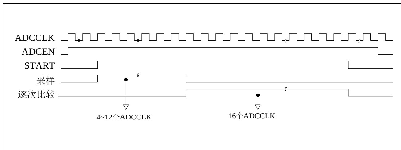
图 27-2 ADC 转换时序图
