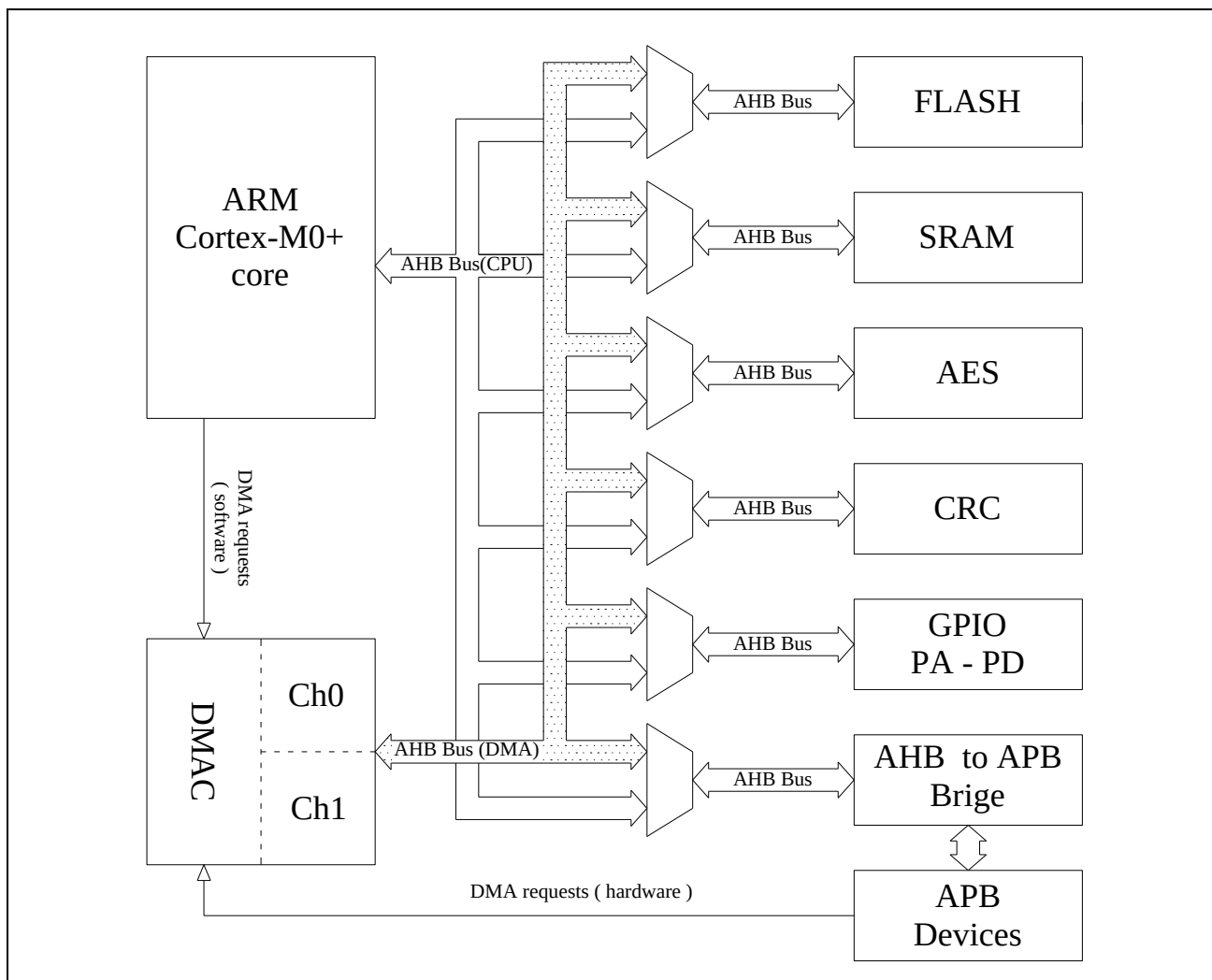
图 13-1 功能框图
