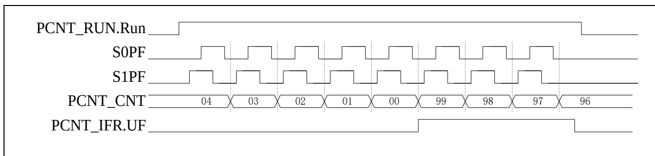
图 20-7 双通道正交脉冲计数模式减计数波形
