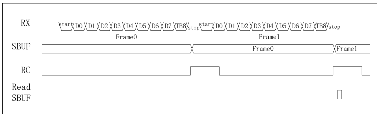
图 21-13 接收缓存
