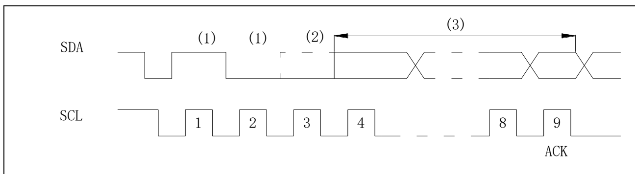
图 7-5 I2C 总线上的仲裁
