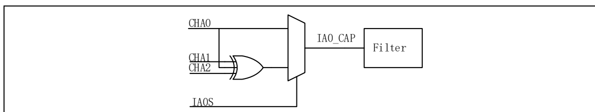
图 14-49 CHA 端口选择
