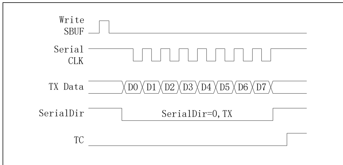
图 22-2 Mode0 发送数据
