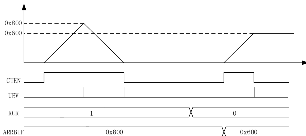
图 14-43 三角波模式单脉冲计数
