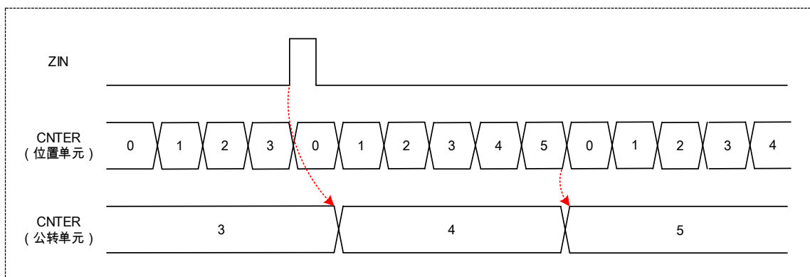
图 17-23 公转模式时 Z 相计数和位置计数器输出混合计数动作
