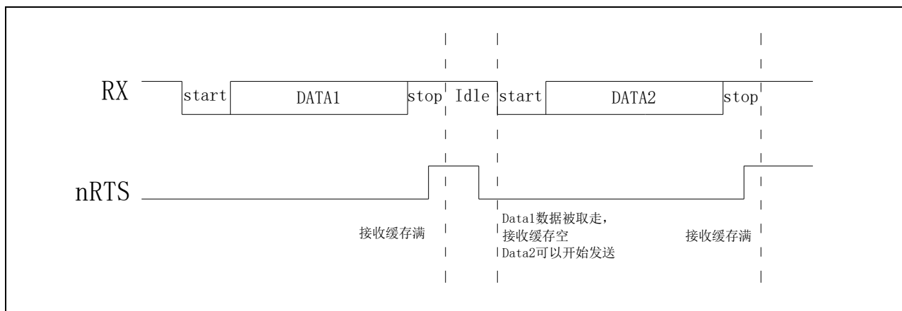
图 22-11 nRTS 硬件流控信号
