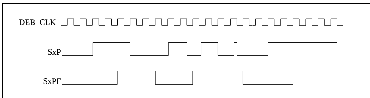
图 20-8 脉冲宽度滤波波形
