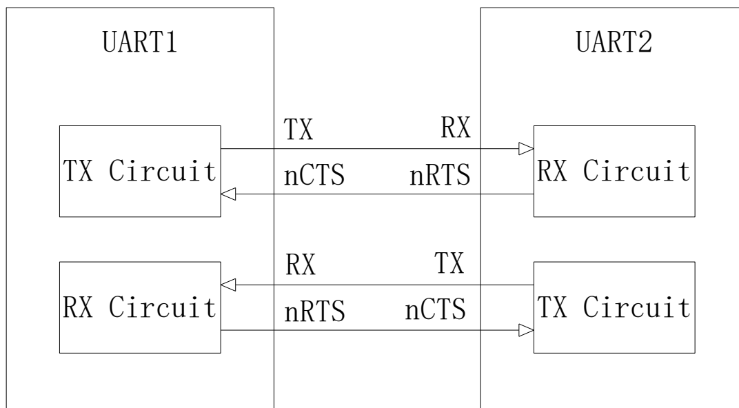
图 21-10 UART 硬件流控
