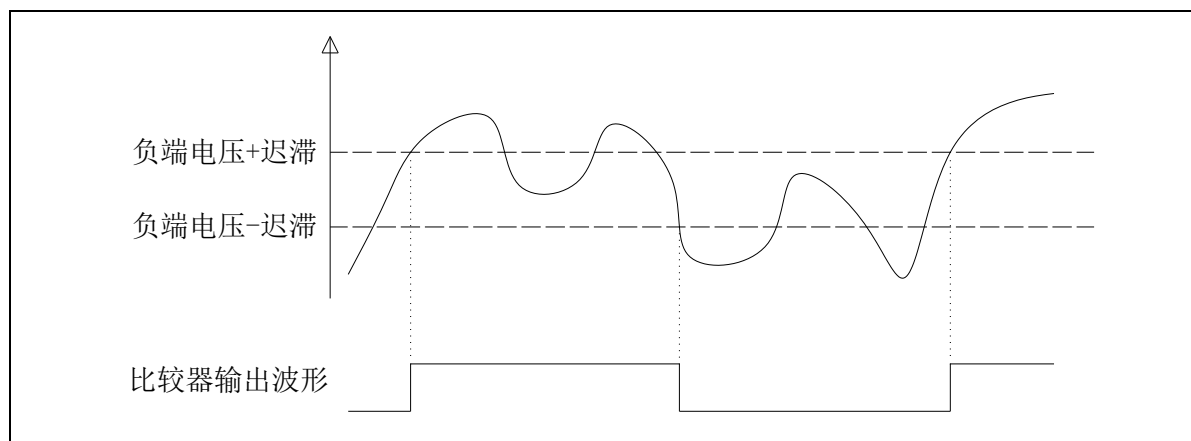
图 28-3 VC 迟滞功能
