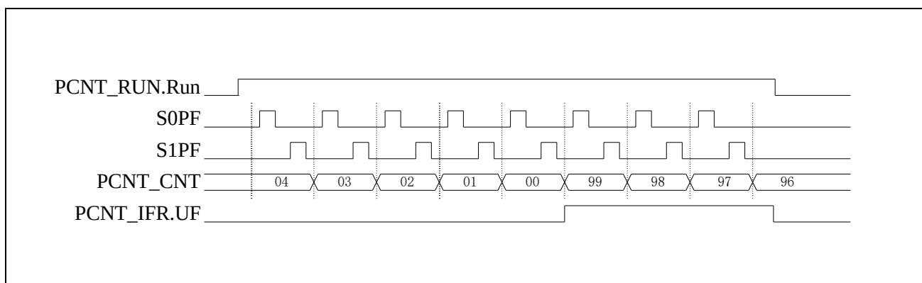
图 20-5 双通道非交脉冲计数模式减计数波形
