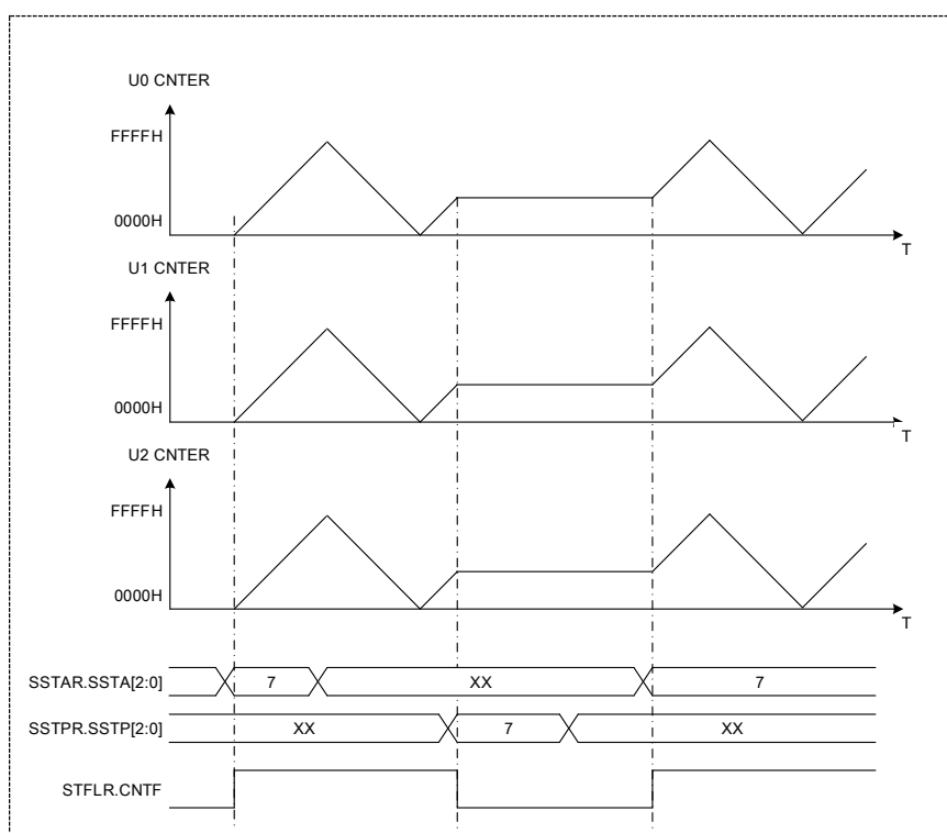
图 17-7 软件同步动作
