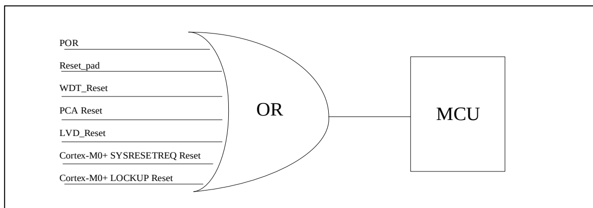
图 4-1 复位来源示意图
