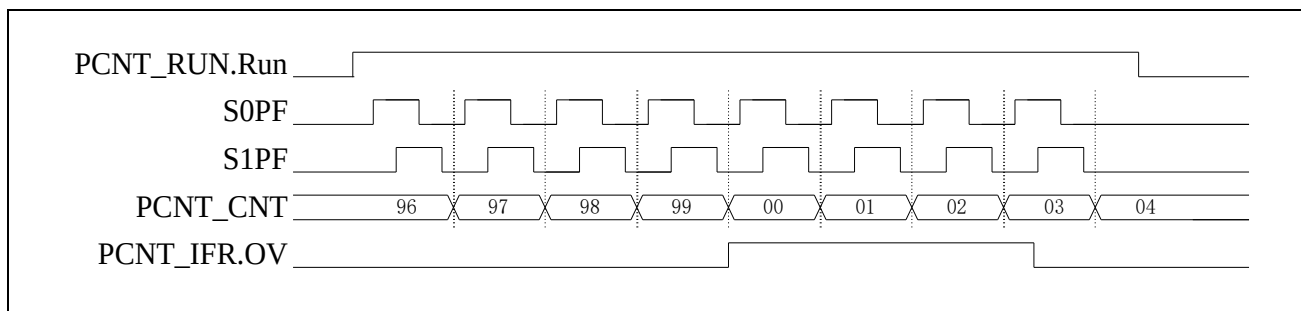
图 20-6 双通道正交脉冲计数模式加计数波形
