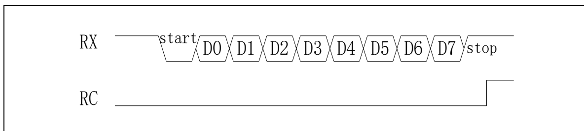
图 22-5 Mode1 接收数据
