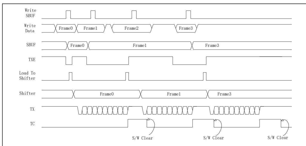
图 21-14 发送缓存
