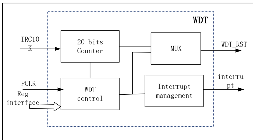
图 19-1 WDT 整体框图
