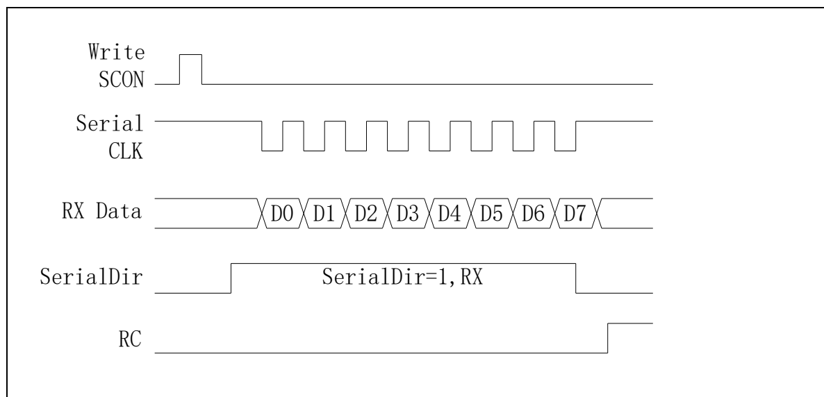
图 22-3 Mode0 接收数据
