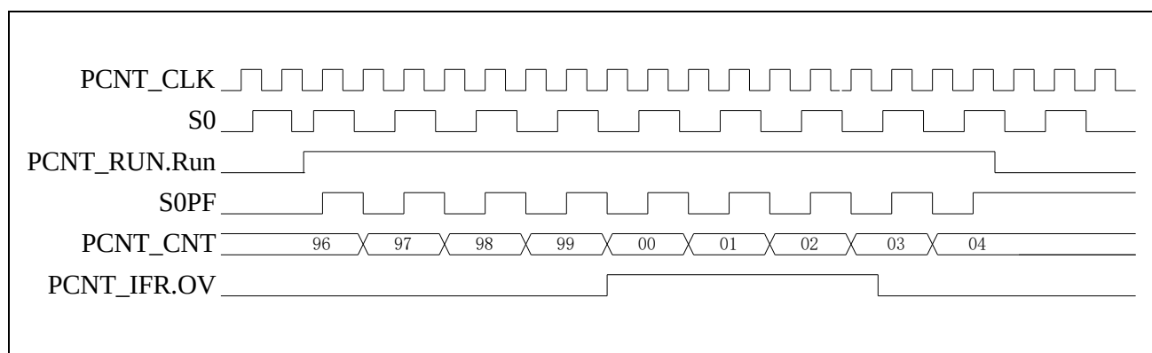
图 20-2 单通道脉冲计数模式加计数波形
