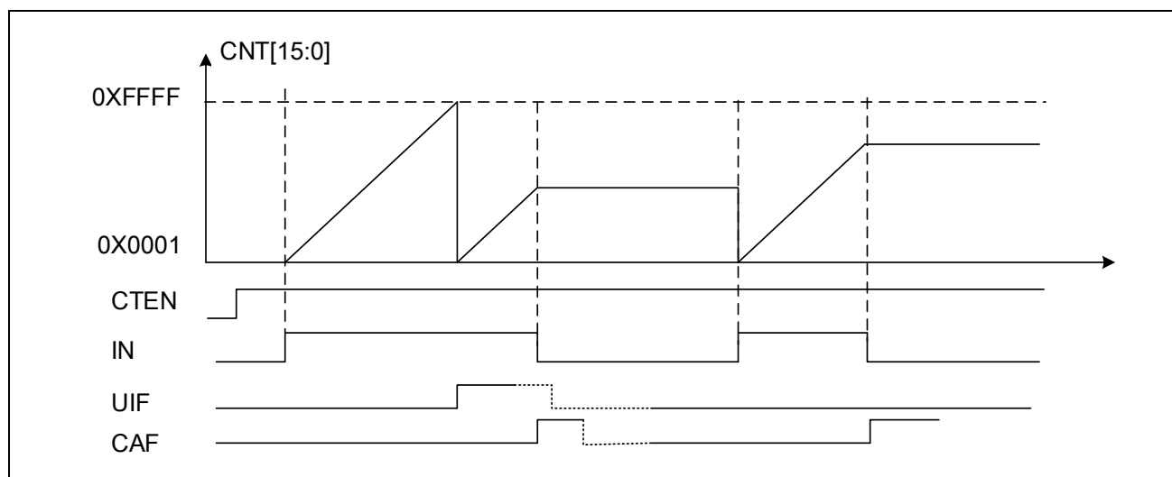
图 14-10 高电平脉冲宽度测量
