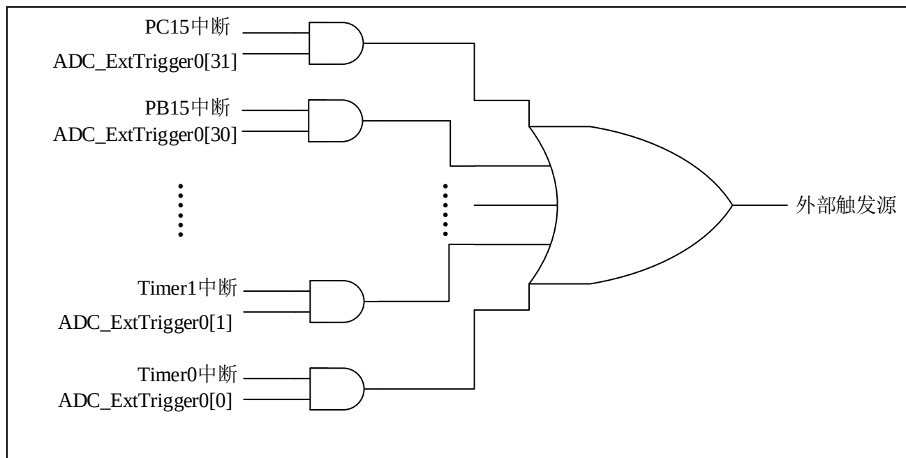
图 27-7 ADC 单次转换或顺序扫描转换外部触发源示意图
