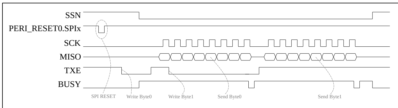
图 8-2 从机发送示意图
