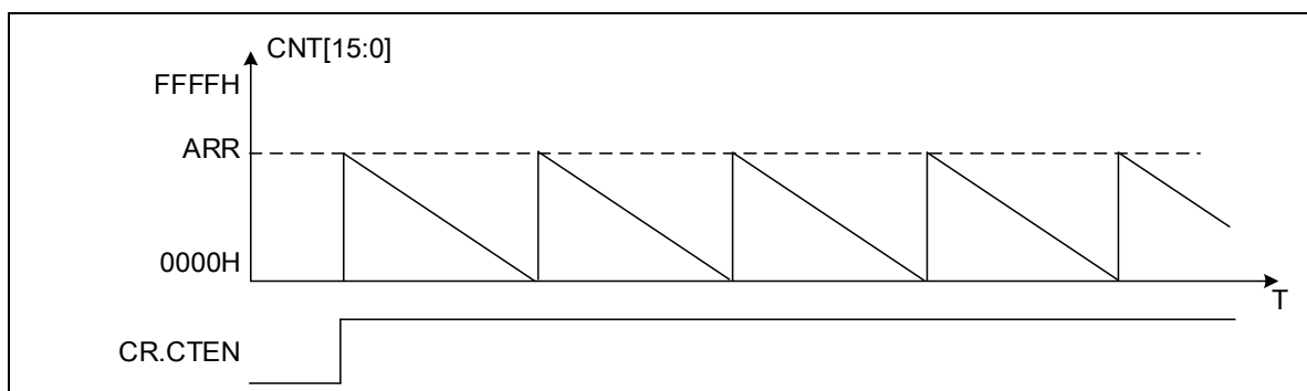
图 14-20 边沿对齐计数器波形(DIR =1)
