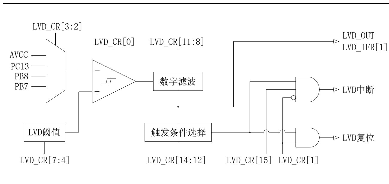
图 29-1 LVD 框图
