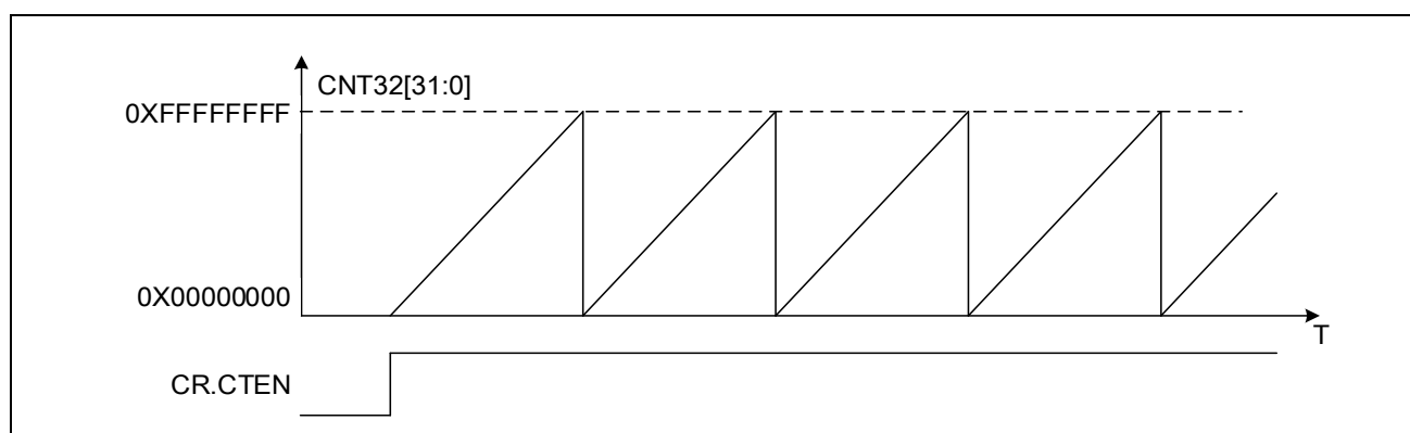
图 14-6 32位自由计数波形
