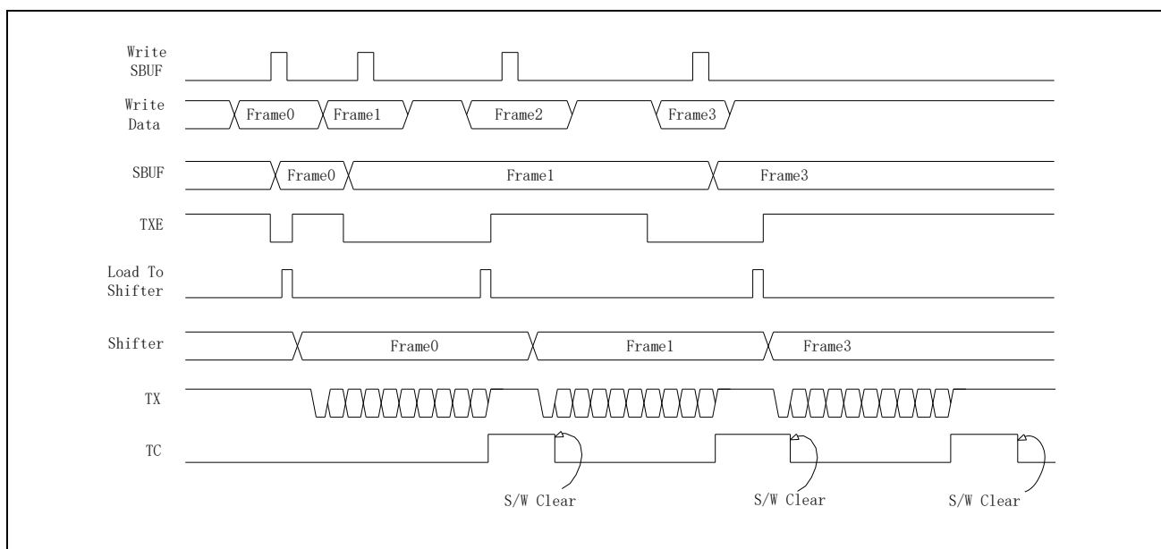
图 22-14 发送缓存
