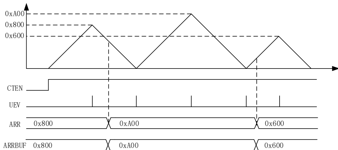
图 14-25 三角波模式下缓存无效
