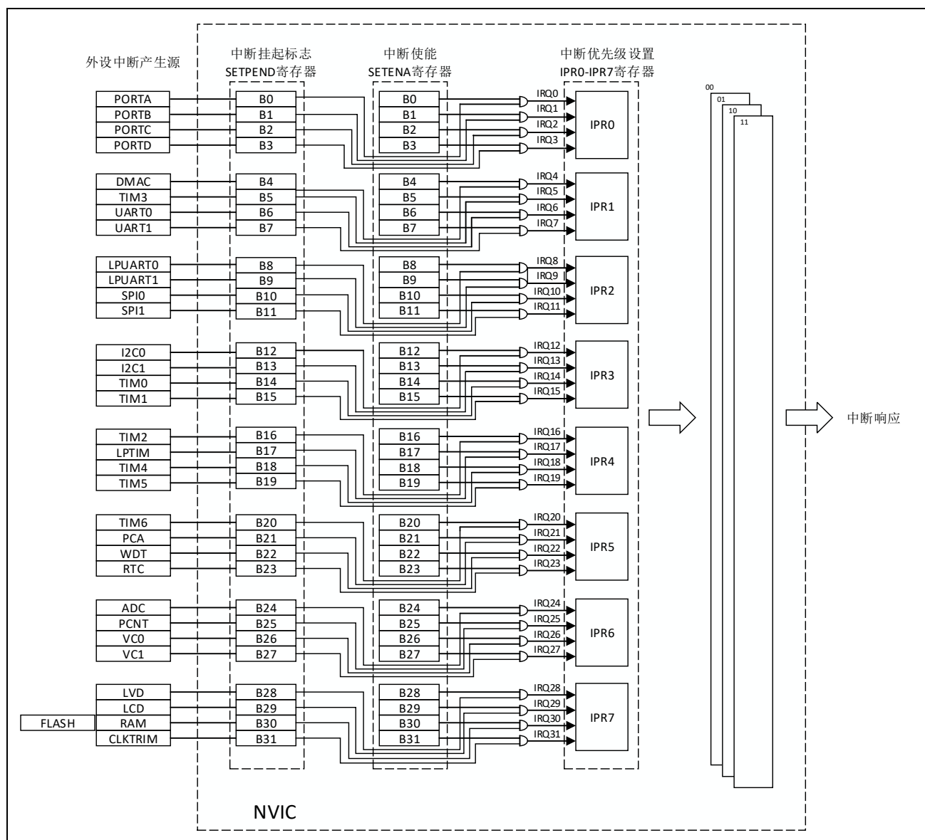
图 5-7 中断结构图
