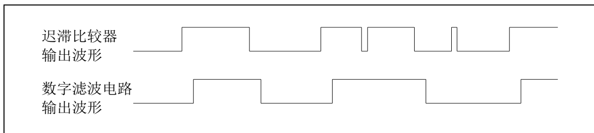
图 29-3 LVD 滤波输出
