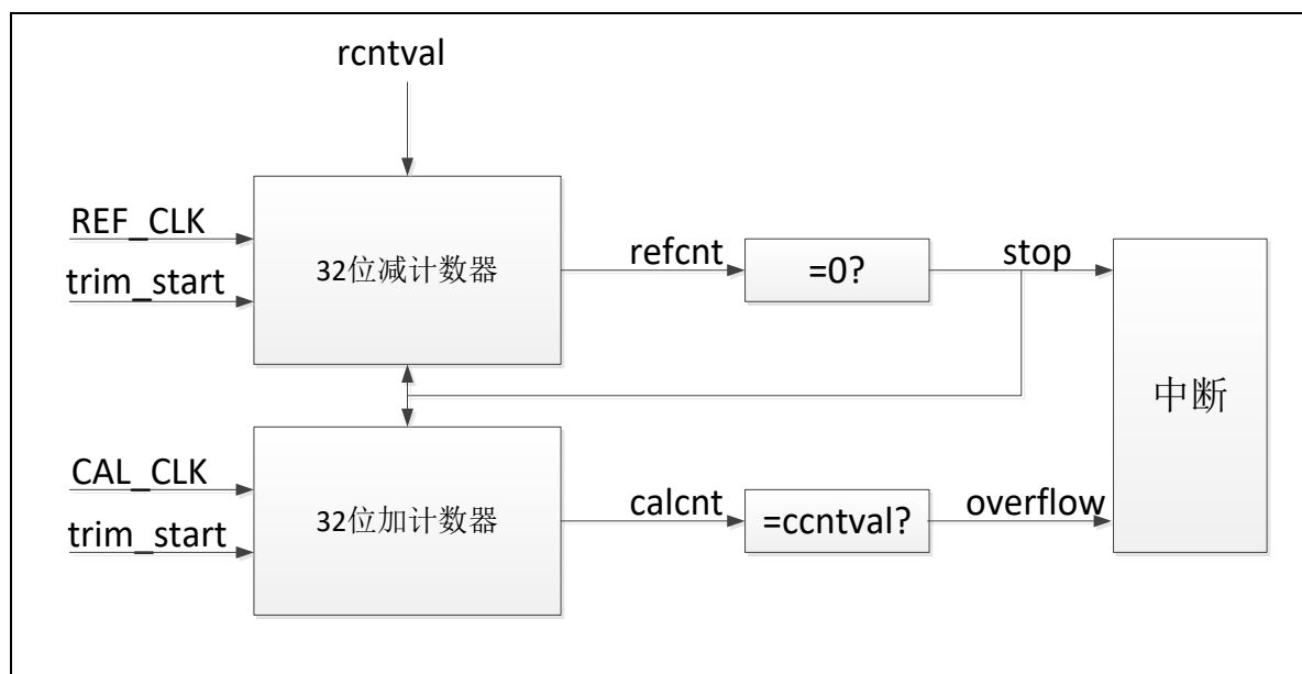
图 9-2 时钟校准模块硬件示意图
