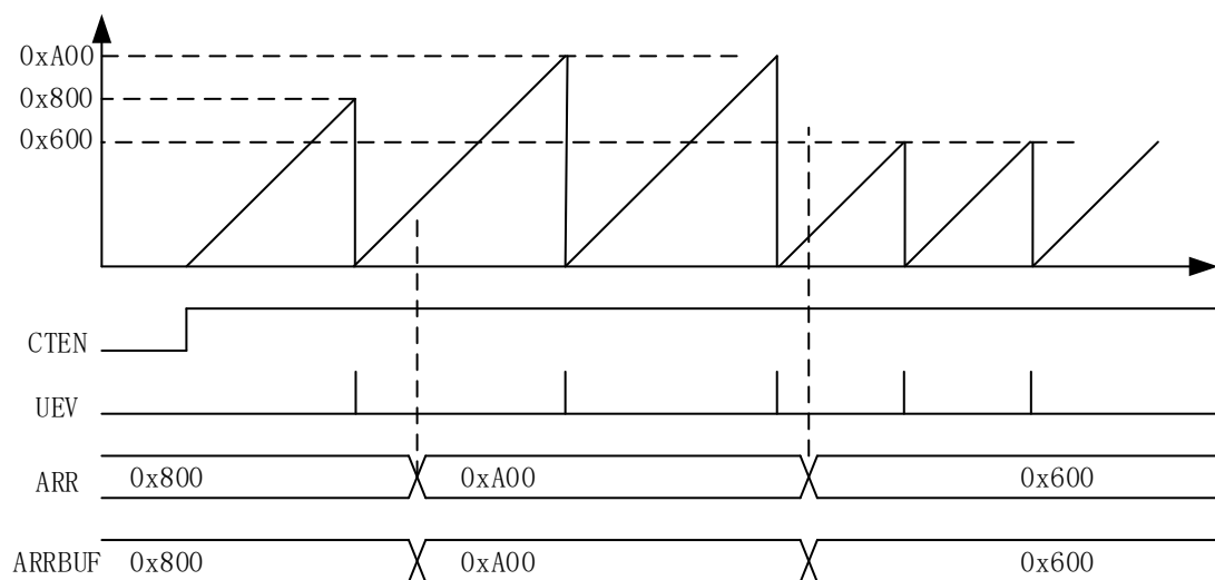
图 14-27 锯齿波模式下上计数缓存无效
