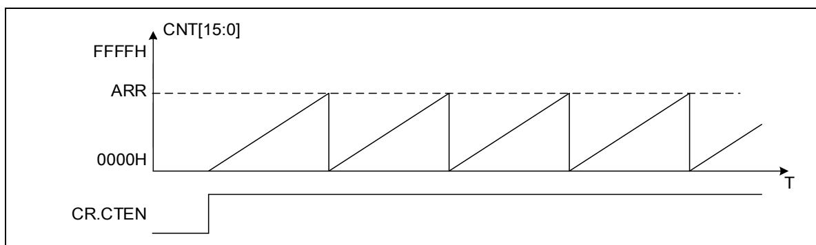
图 14-21 边沿对齐计时器波形(DIR =0)
