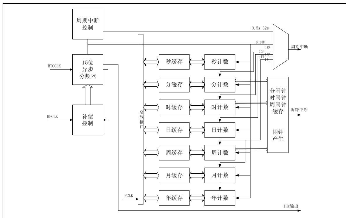
图 18-1 RTC 框图
