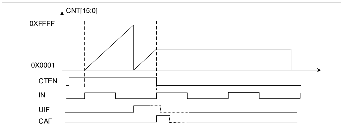
图 14-13 上升沿到上升沿周期测量单次模式
