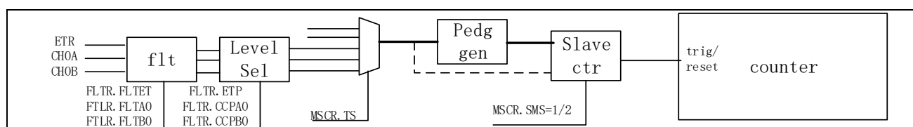
图 14-53 触发和复位功能
