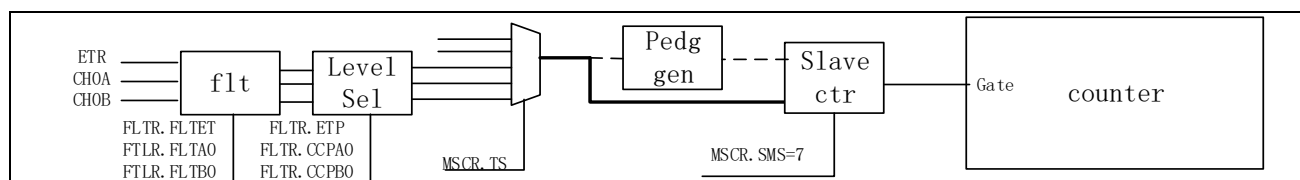
图 14-52 门控功能
