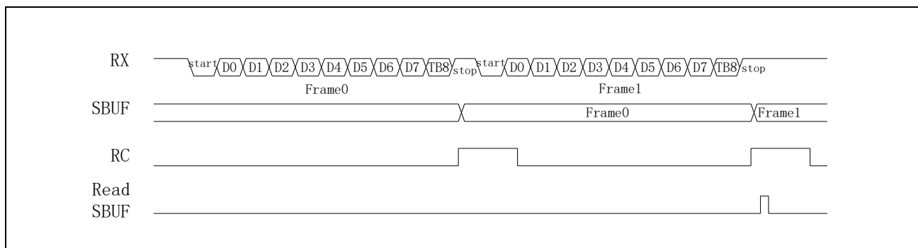
图 22-13 接收缓存
