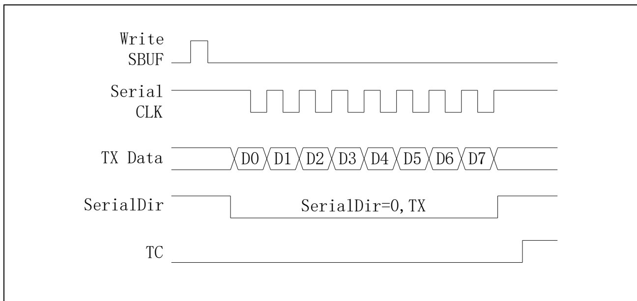
图 21-2 Mode0 发送数据
