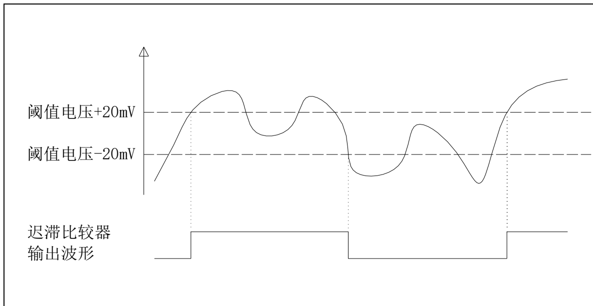
图 29-2 LVD 迟滞响应
