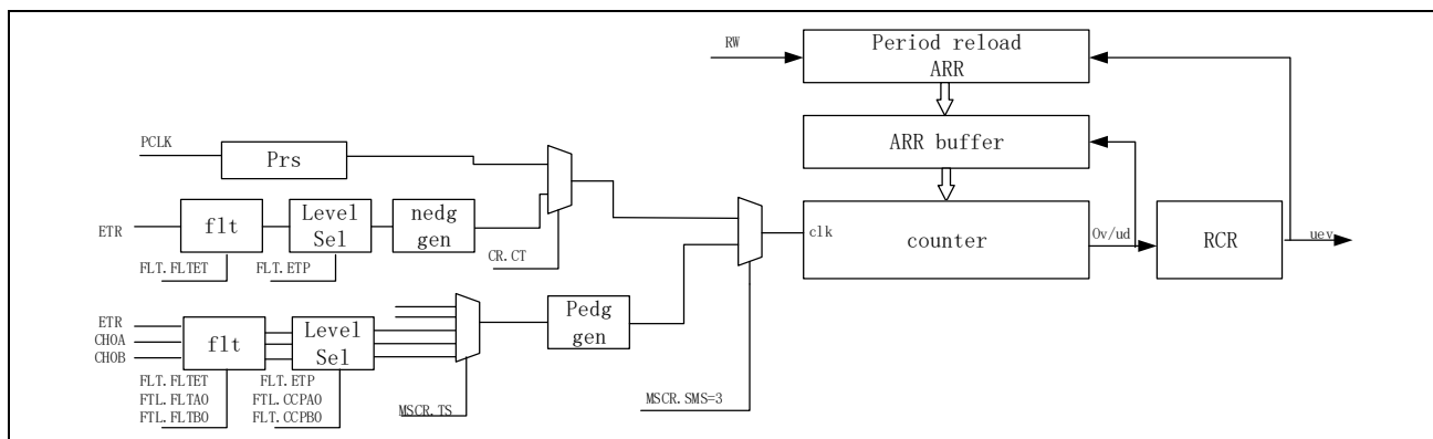
图 14-14 计数器框图
