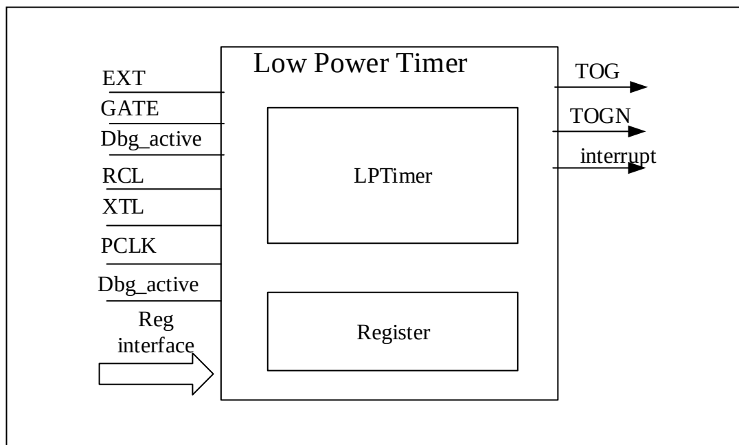
图 15-1 LPTimer 框图
