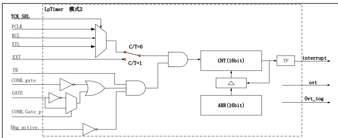
图 15-3 LPTimer 模式 2
