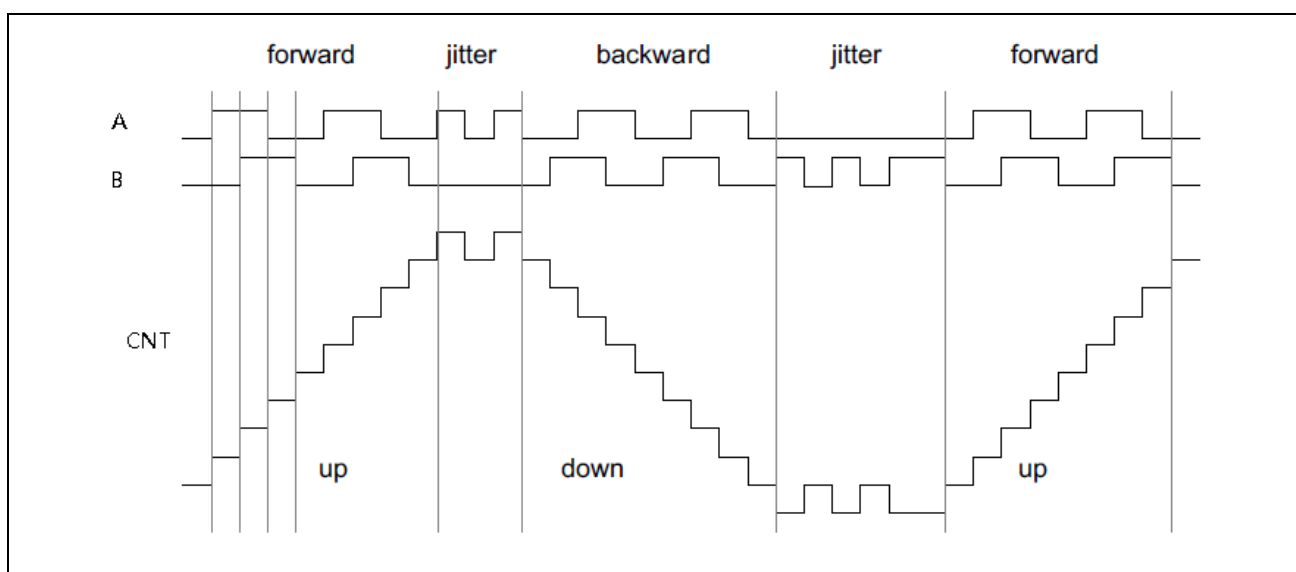
图 14-54 编码计数
