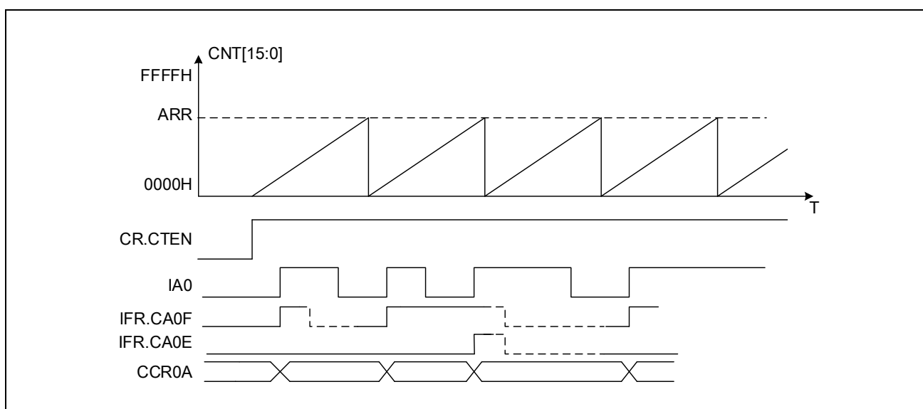
图 14-48 捕获时序图
