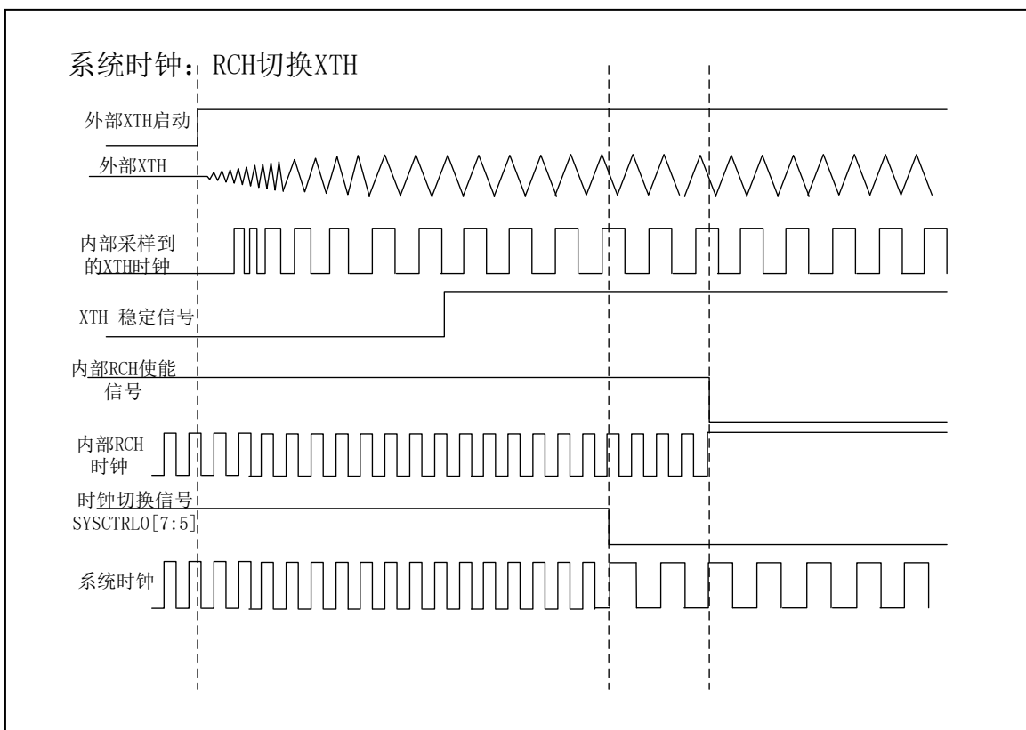
图 3-3 时钟切换示意图
