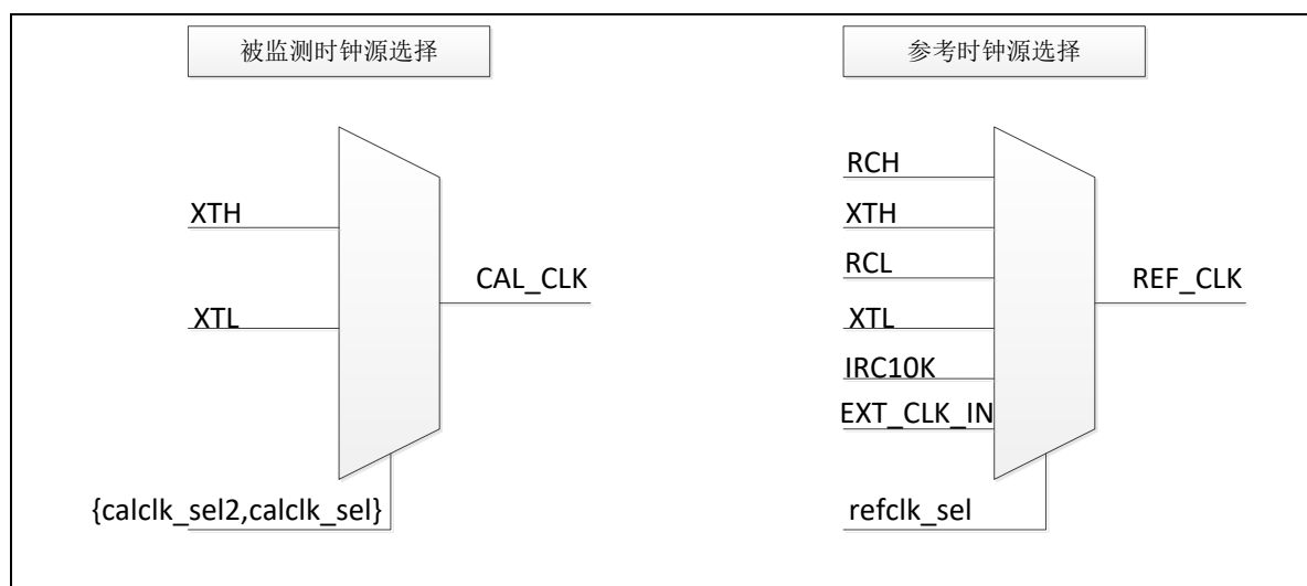
图 9-4 CLKTRIM 时钟选择
