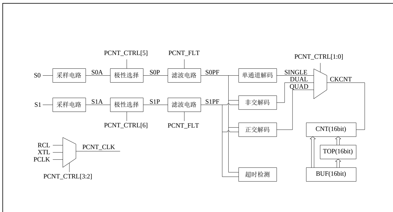
图 20-1 整体框图
