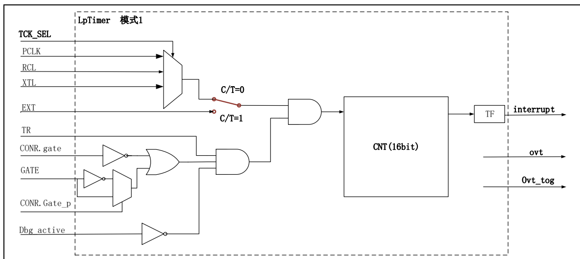
图 15-2 LPTimer 模式 1
