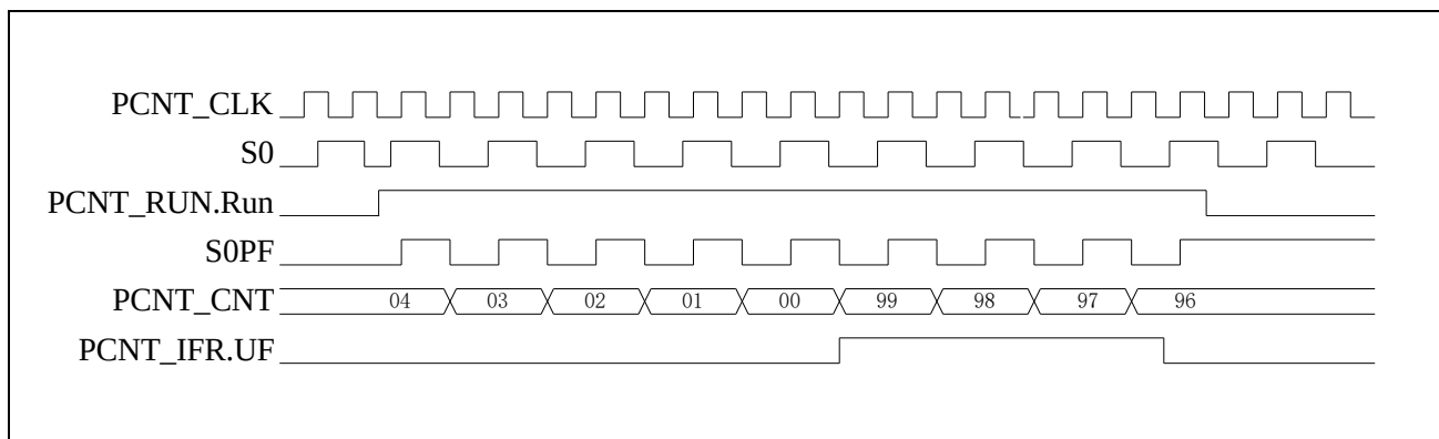
图 20-3 单通道脉冲计数模式减计数波形
