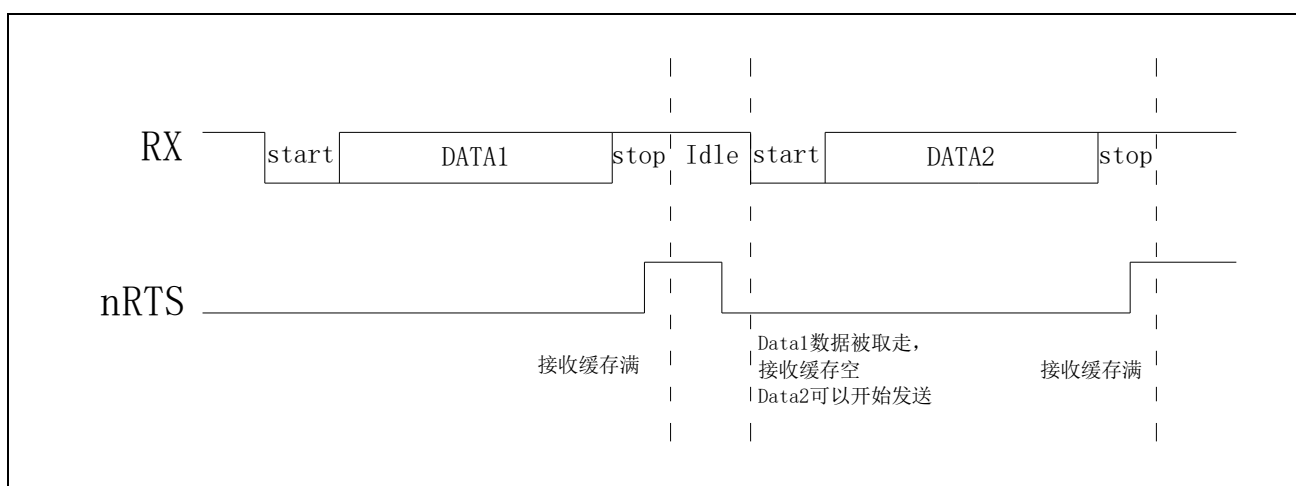
图 21-11 nRTS 硬件流控信号
