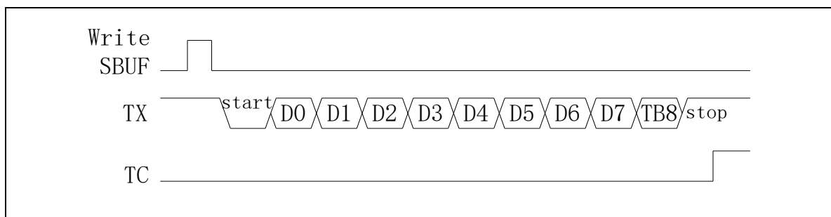
图 22-8 Mode3 发送数据
