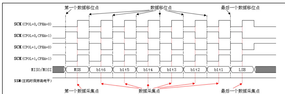
图 8-3 主机模式帧格式
