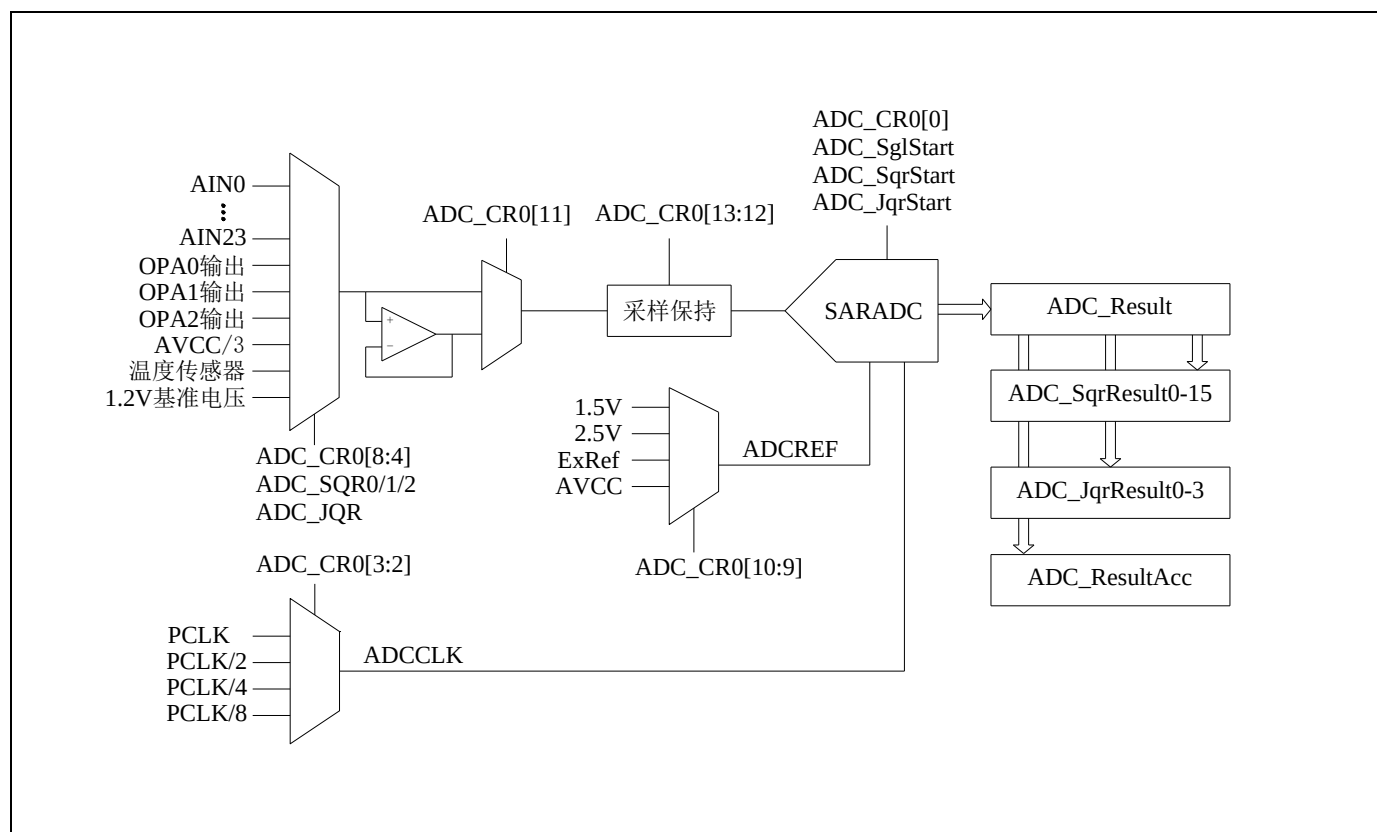
图 27-1 ADC 示意框图
