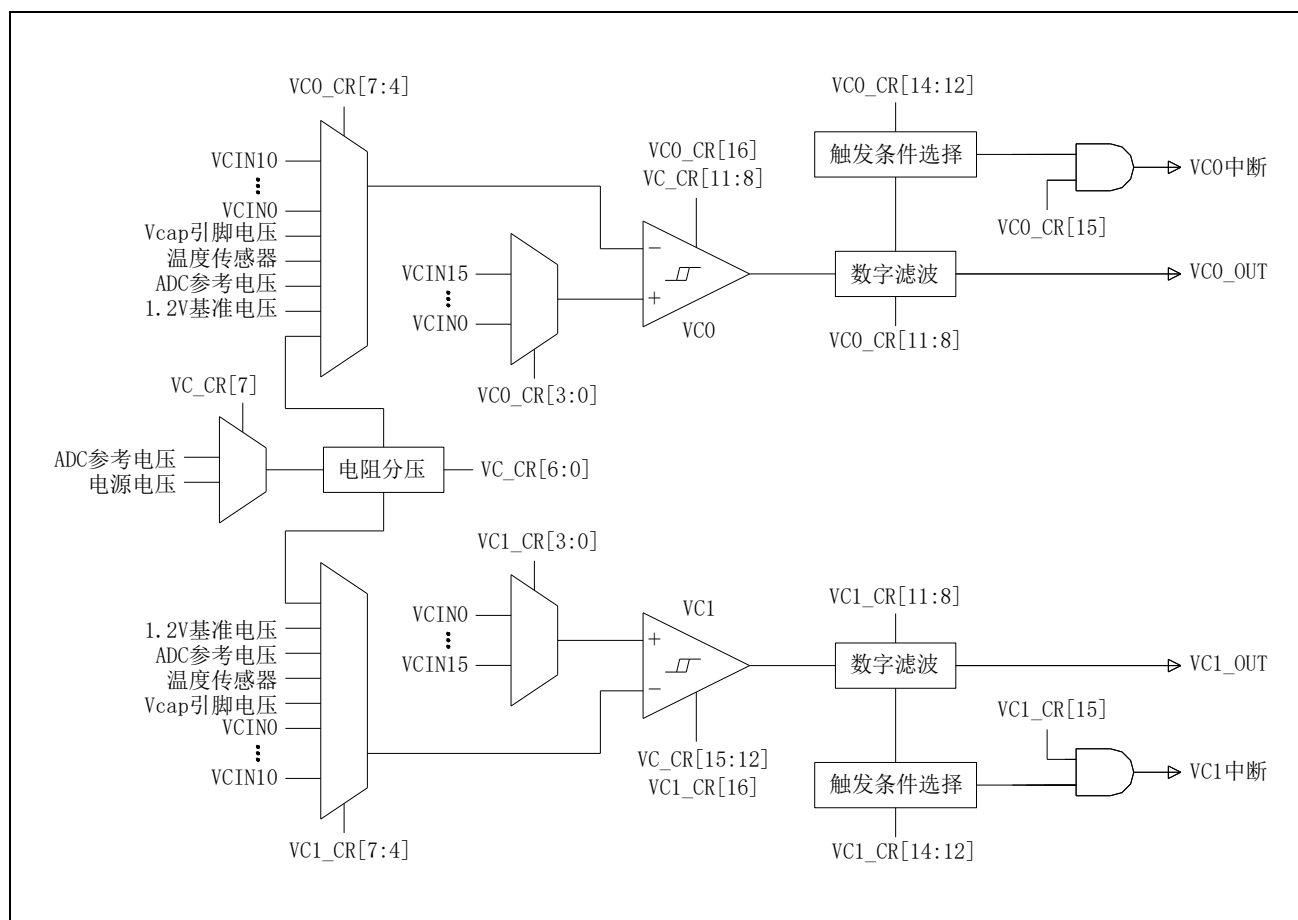
图 28-1 VC 框架图
