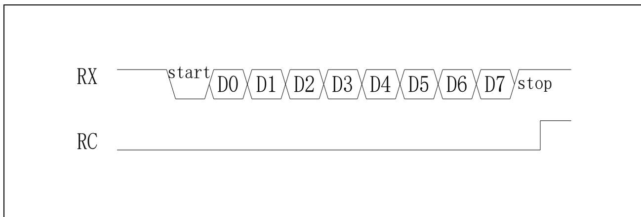
图 21-5 Mode1 接收数据
