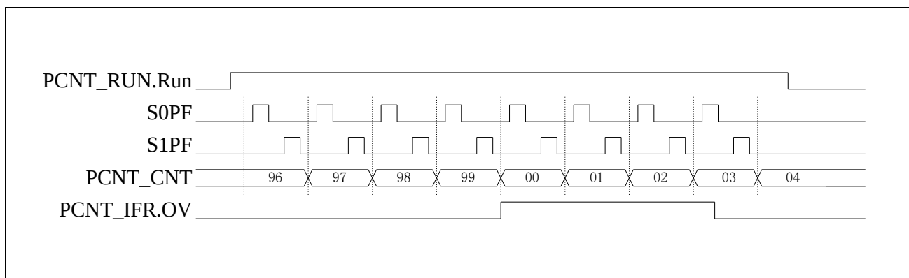
图 20-4 双通道非交脉冲计数模式加计数波形
