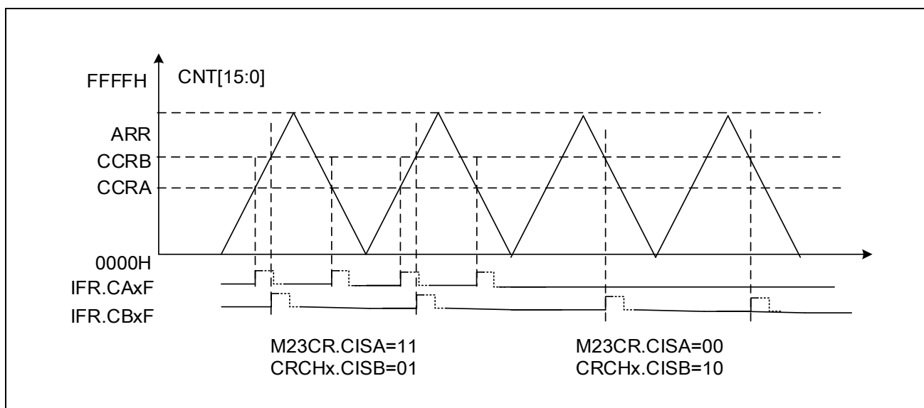
图 14-46 中断示意图
