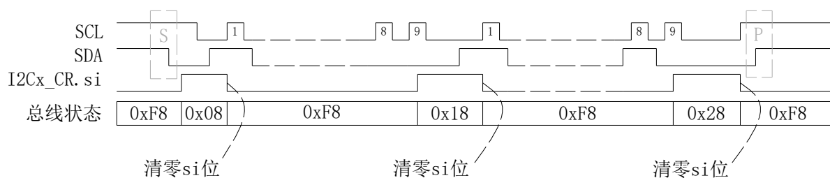
图 7-7 主发送模式数据同步图
