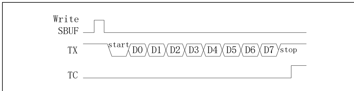
图 22-4 Mode1 发送数据
