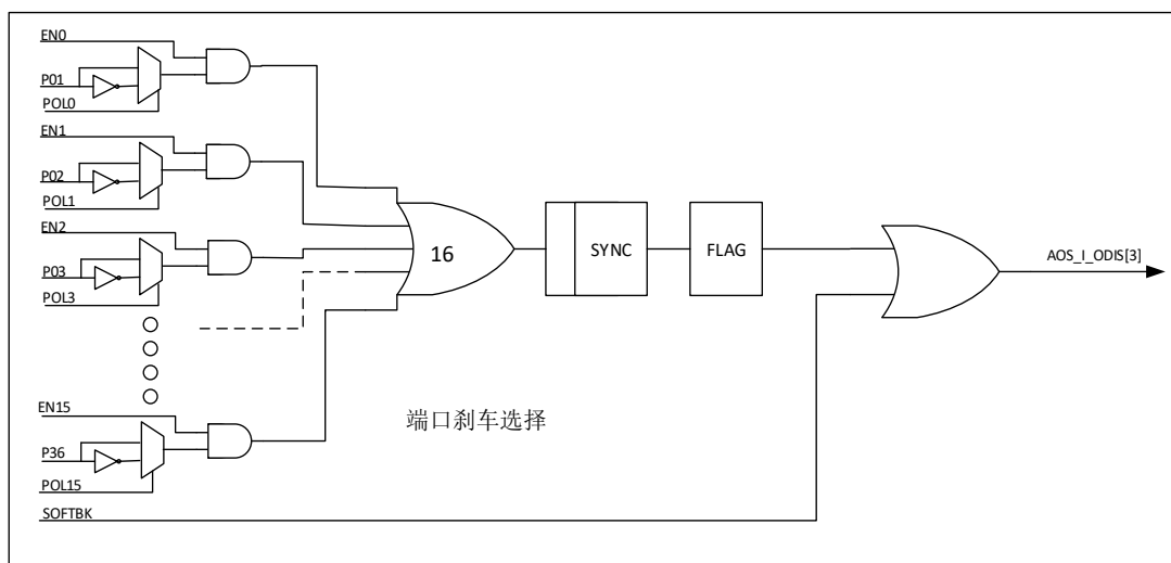
图 17-27 端口刹车与软件刹车示意图
