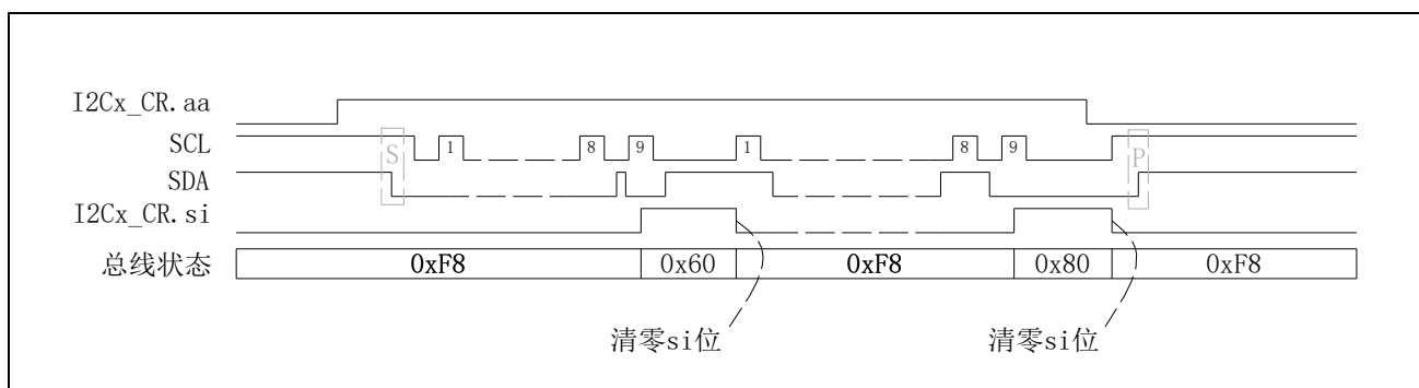
图 7-11 从接收模式数据同步图
