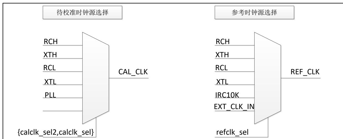
图 9-1 时钟源选择示意图
