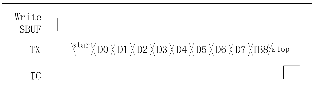
图 21-6 Mode2 发送数据
