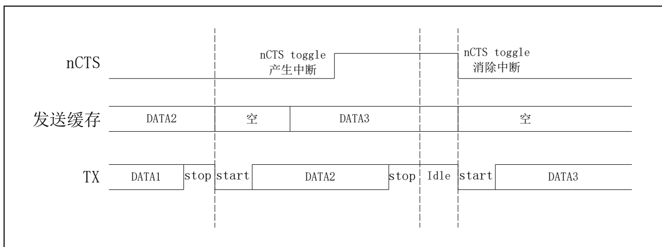
图 22-12 nCTS 硬件流控信号
