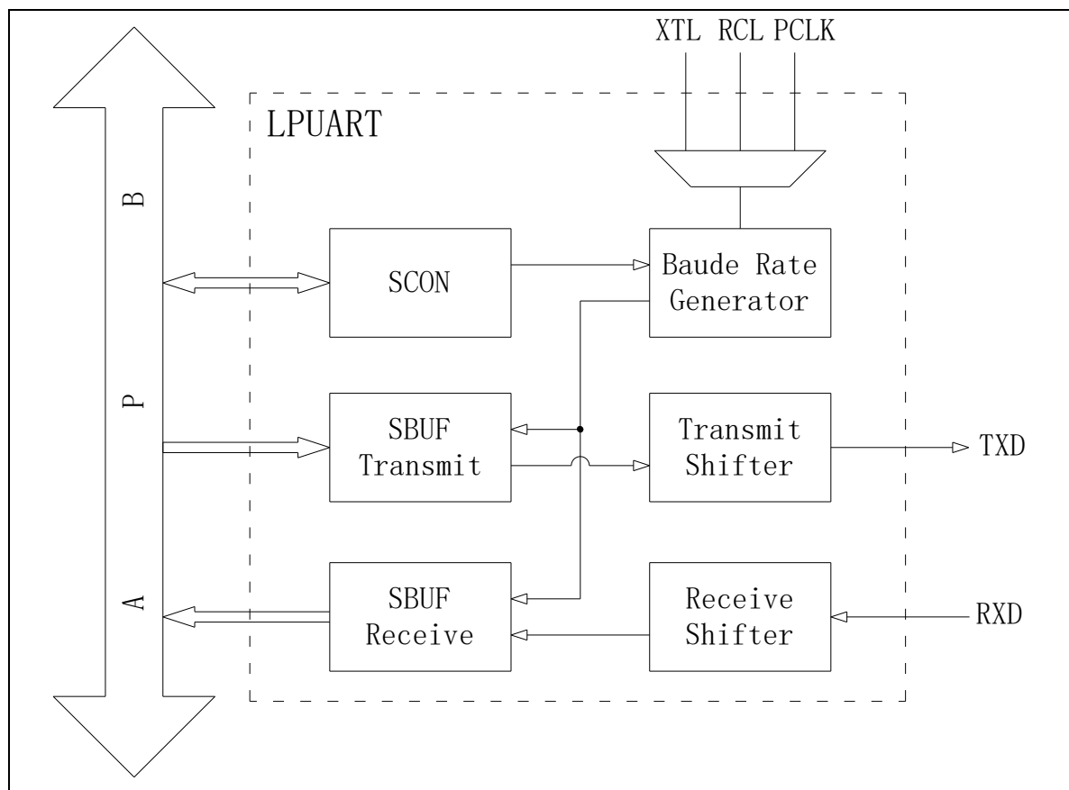
图 22-1 结构框图
