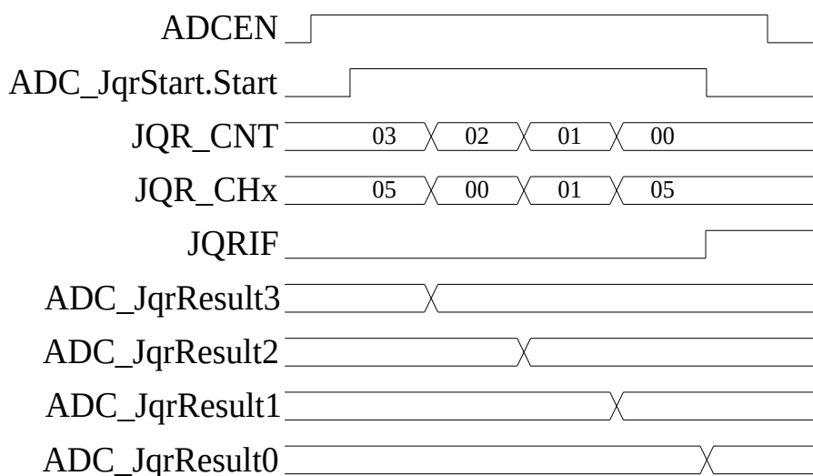
图 27-4 ADC 插队扫描转换过程示例
