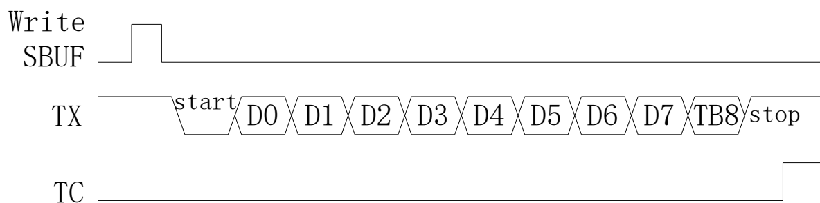
图 21-8 Mode3 发送数据
