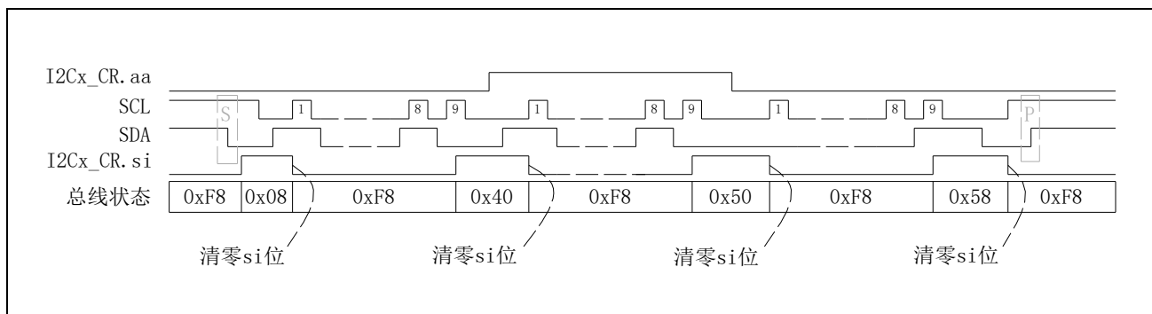
图 7-9 主接收模式数据同步图
