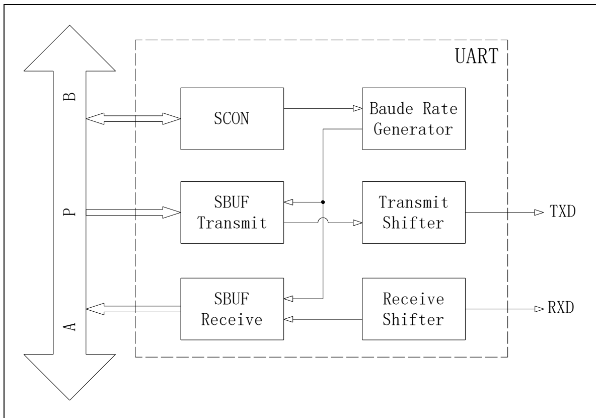
图 21-1 结构框图
