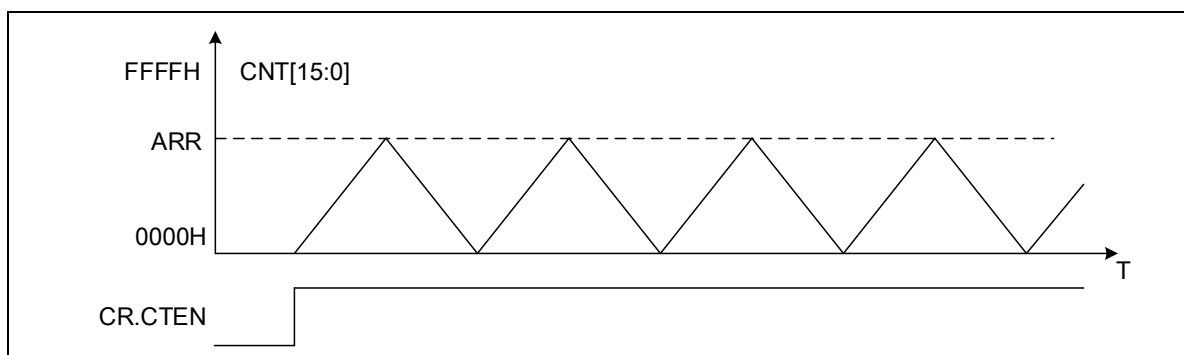
图 14-22 中心对齐计数器波形
