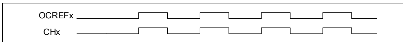
图 14-37 CCPx=0时PWM输出波形
