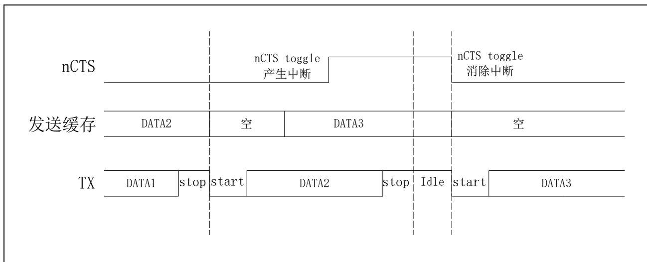
图 21-12 nCTS 硬件流控信号
