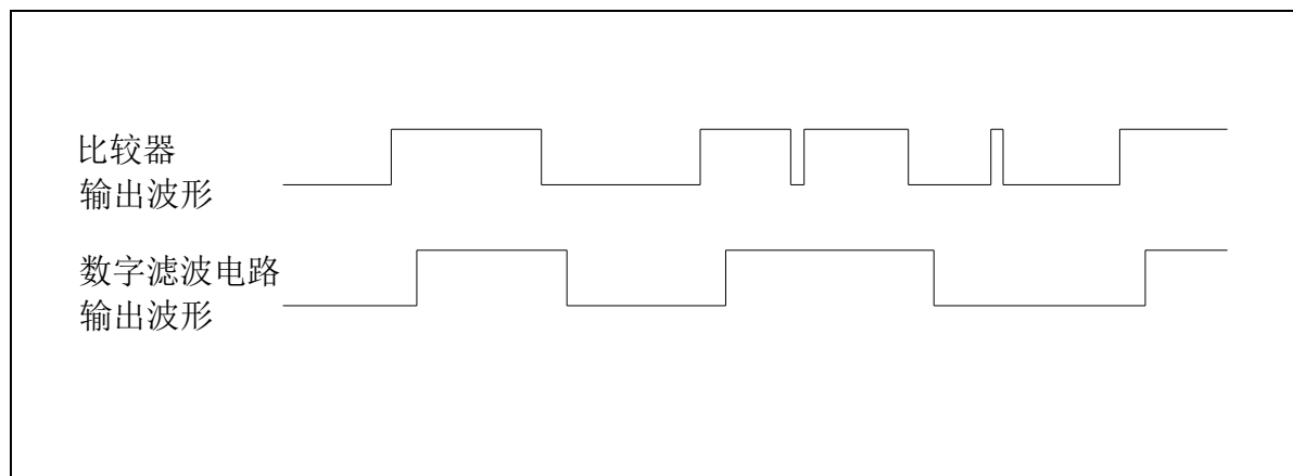
图 28-2 VC 滤波响应时间
