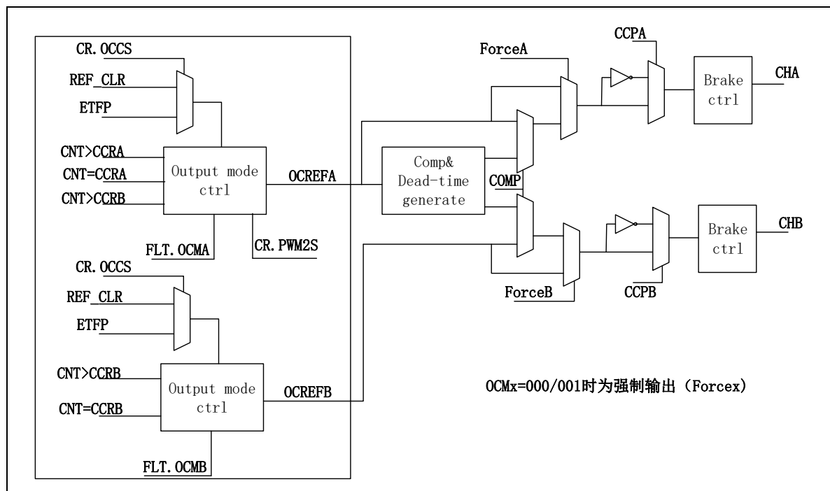
图 14-31 OCREF 输出框图
