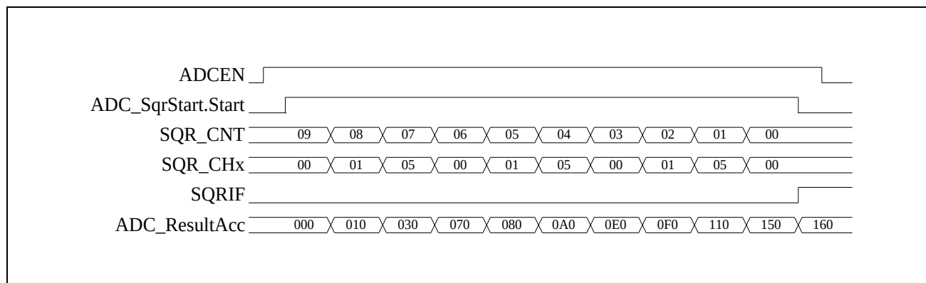
图 27-6 ADC 连续转换累加过程示例
