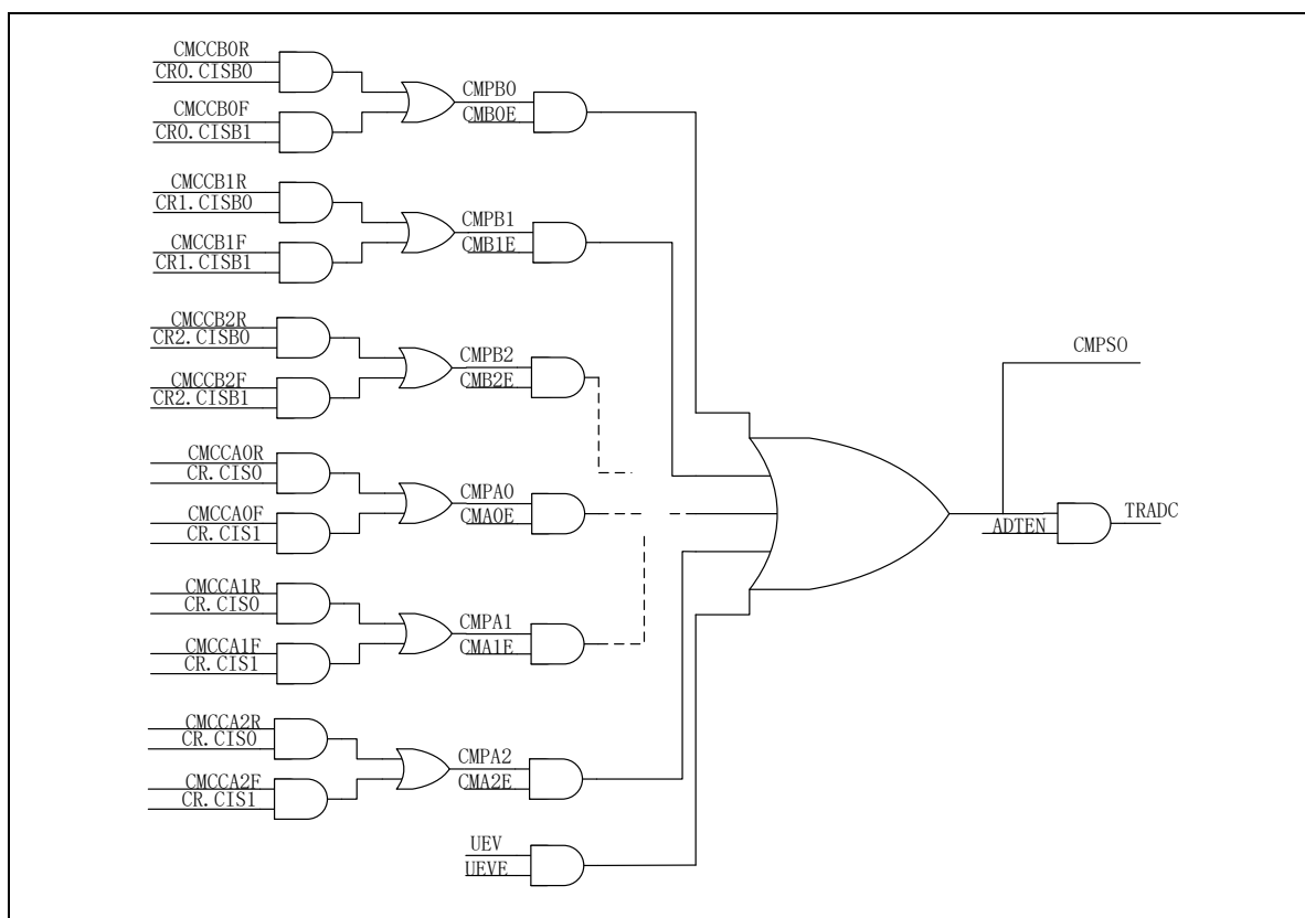
图 14-55 ADC 触发
